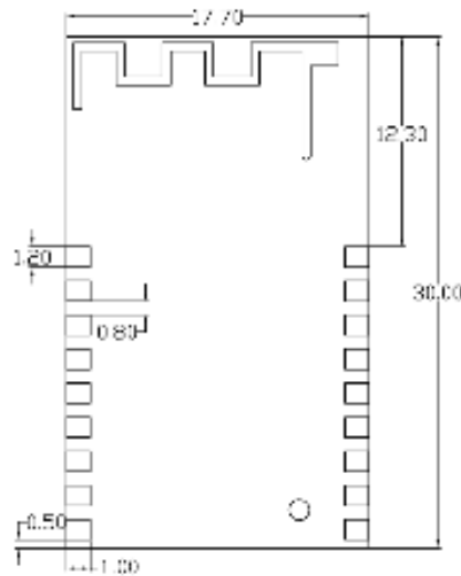
Fig 3 - Module Dimensions
