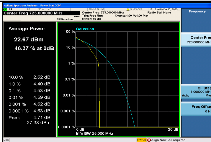
Band28-10MHz-QPSK-27410-1RB#0
