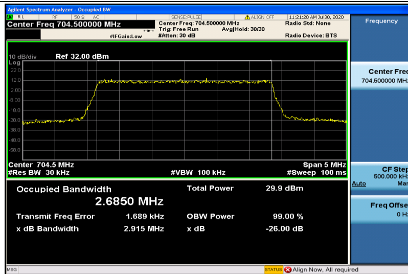
Band28-3MHz-QPSK-27225-15RB#0-2.6850
