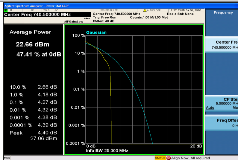
Band28-15MHz-QPSK-27585-1RB#0
