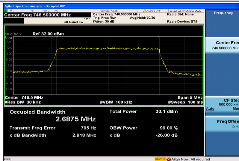
Band28-3MHz-QPSK-27645-15RB#0-2.6875
