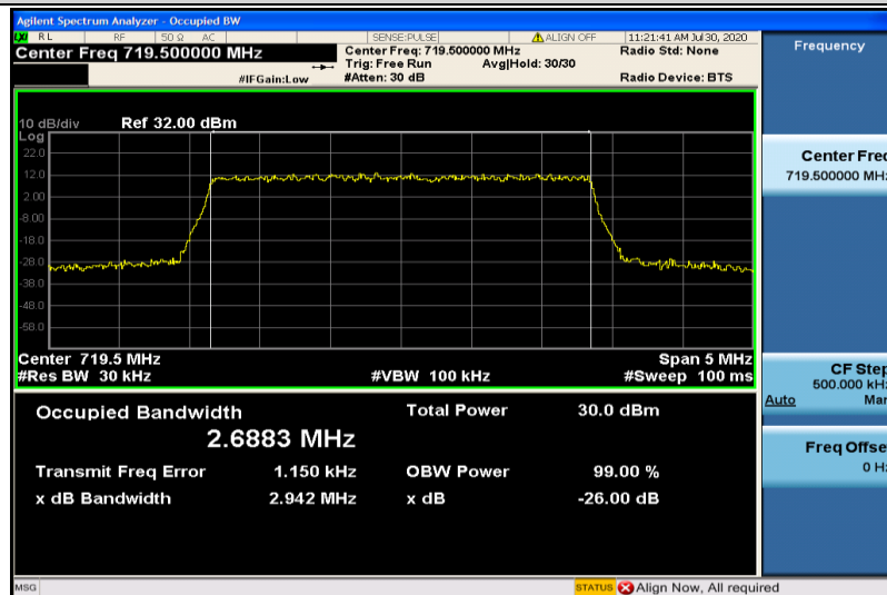
Band28-3MHz-QPSK-27375-15RB#0-2.6883
