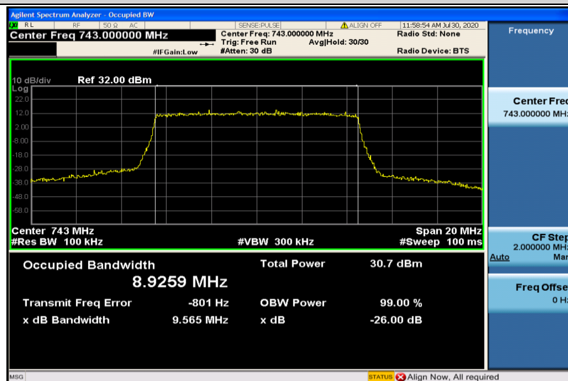
Band28-10MHz-QPSK-27610-50RB#0-8.9259
