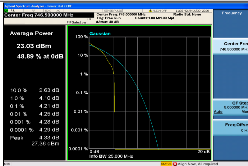
Band28-3MHz-QPSK-27645-1RB#0
