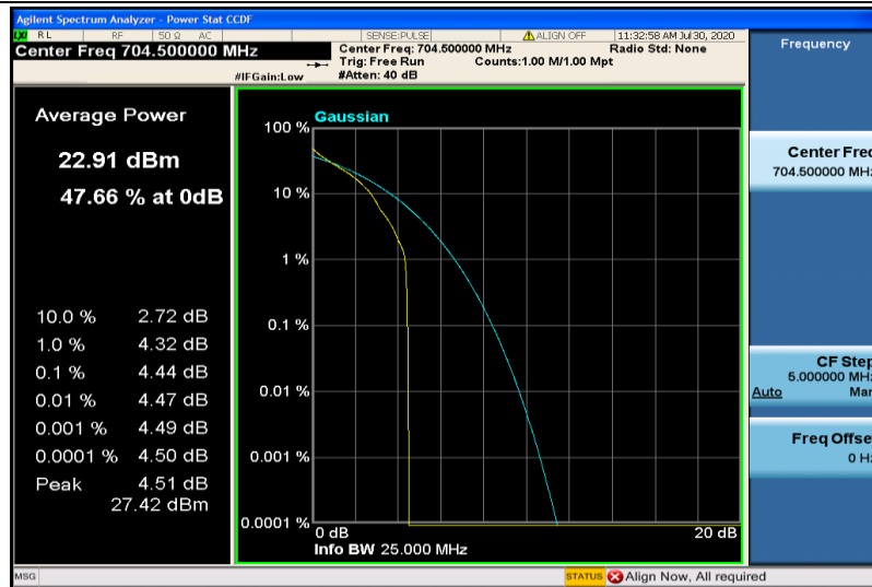
Band28-3MHz-QPSK-27225-1RB#0
