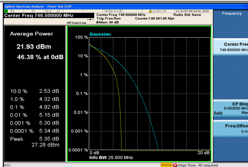
Band28-3MHz-QPSK-27645-15RB#0
