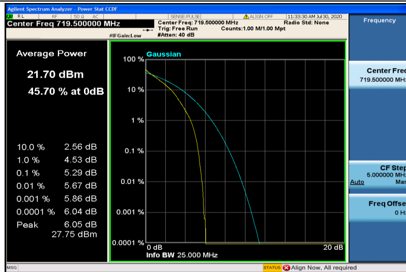
Band28-3MHz-QPSK-27375-15RB#0
