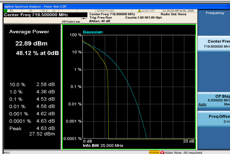
Band28-3MHz-QPSK-27375-1RB#0
