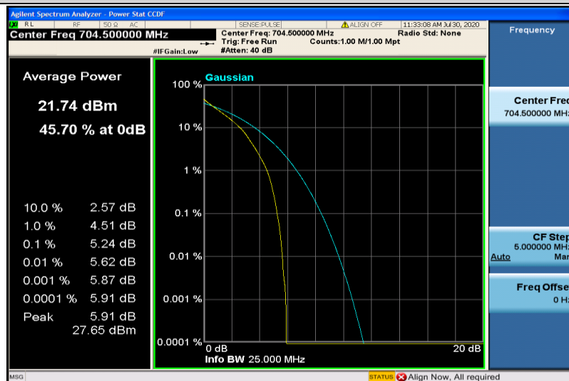
Band28-3MHz-QPSK-27225-15RB#0
