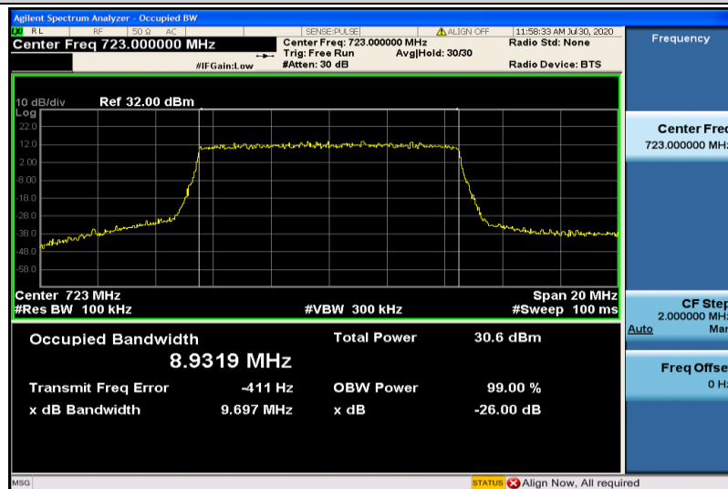
Band28-10MHz-QPSK-27410-50RB#0-8.9319
