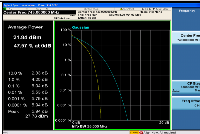
Band28-10MHz-QPSK-27610-50RB#0
