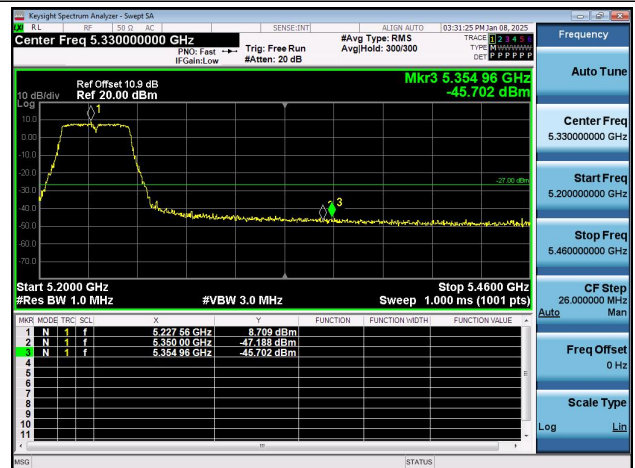
11AC80SISO-Ant1-5210-PASS
