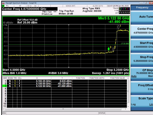
11AX80SISO-Ant2-5210-PASS
