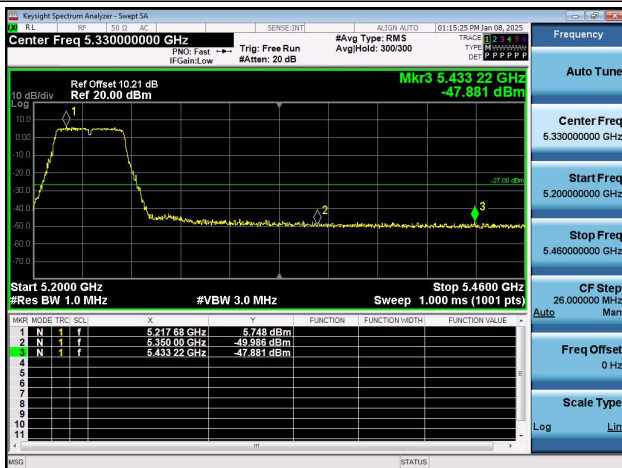
11AC80SISO-Ant1-5210-PASS
