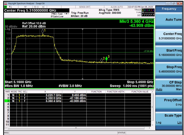
11AX80SISO-Ant2-5210-PASS
