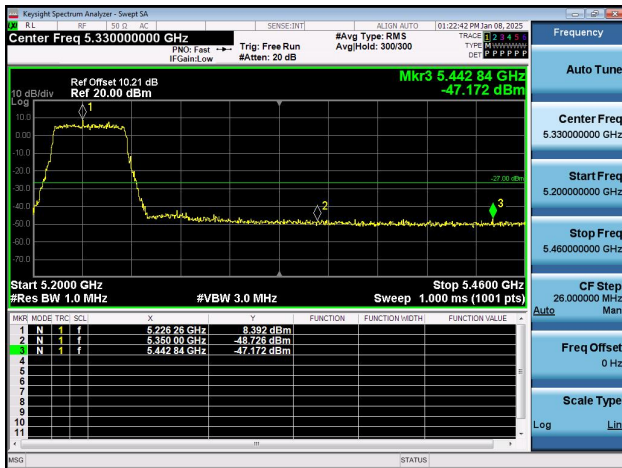
11AX80SISO-Ant1-5210-PASS
