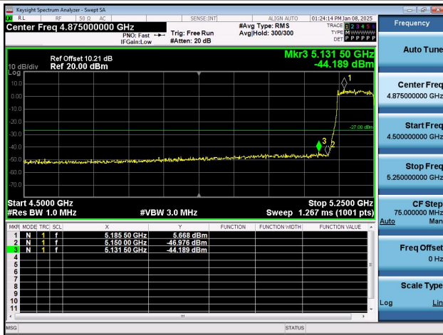
11AX80SISO-Ant2-5210-PASS
