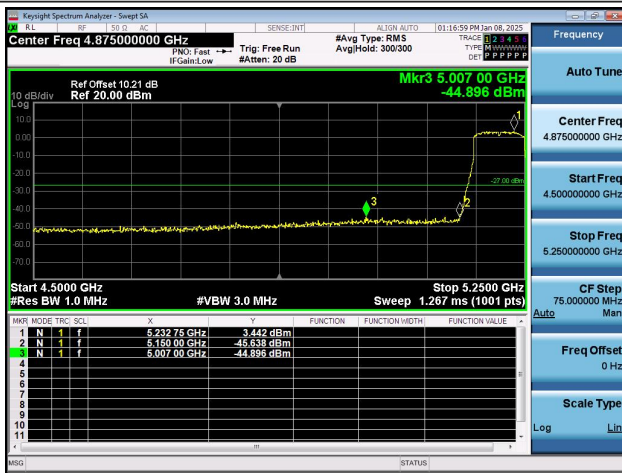
11AC80SISO-Ant2-5210-PASS
