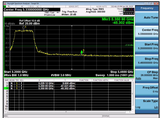
11AX80SISO-Ant1-5210-PASS
