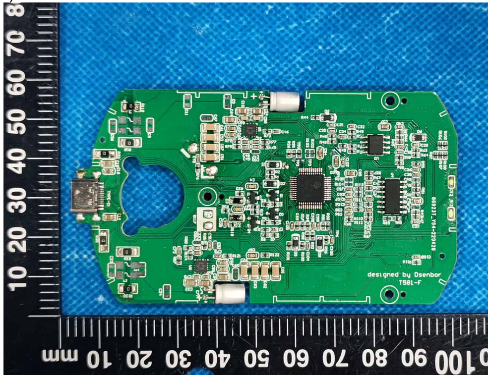
6) EUT Photo
