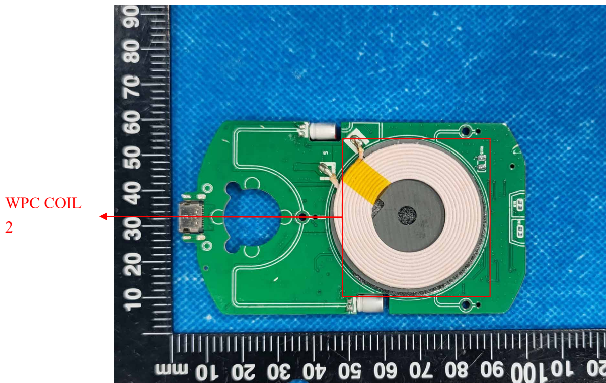
4) EUT Photo
