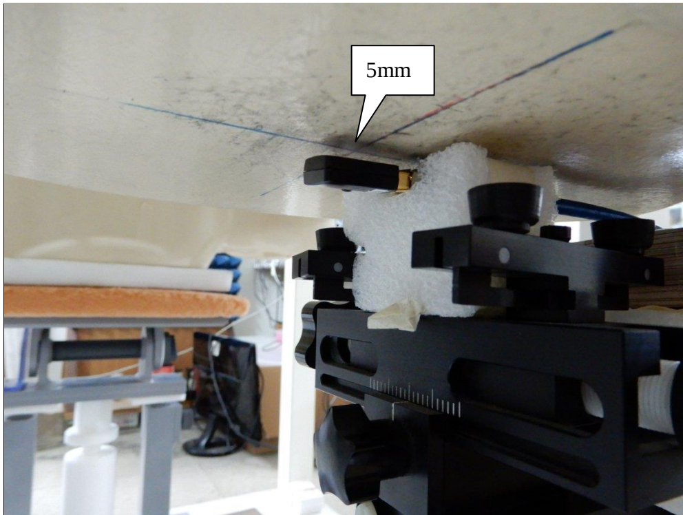
EUT Back
