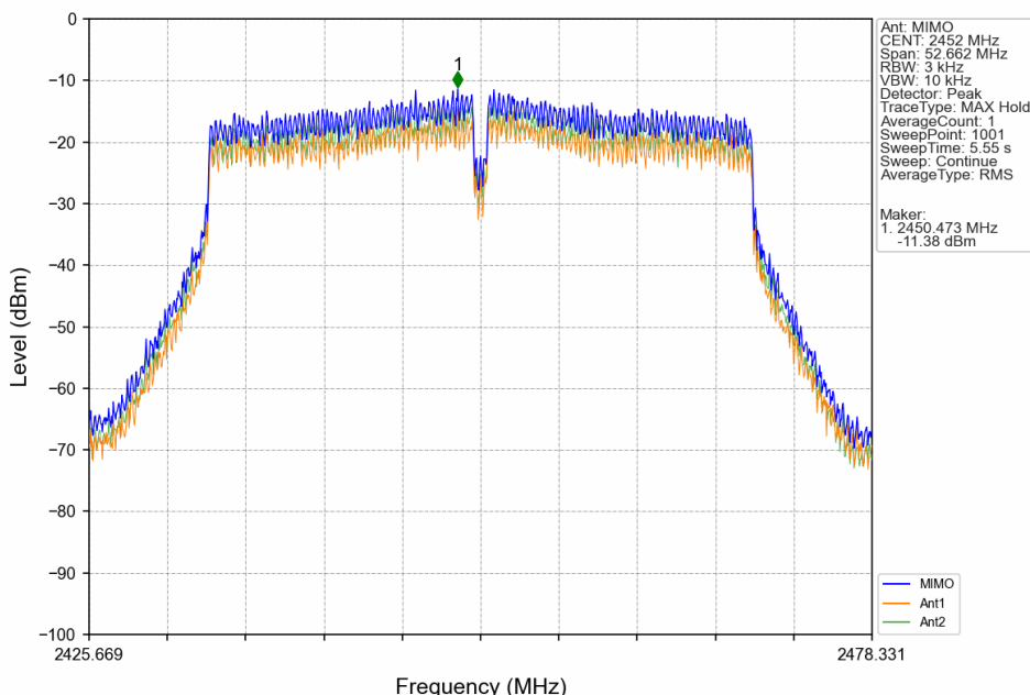
802.11n(HT40)_HCH_2452MHz_MIMO_NTNV
