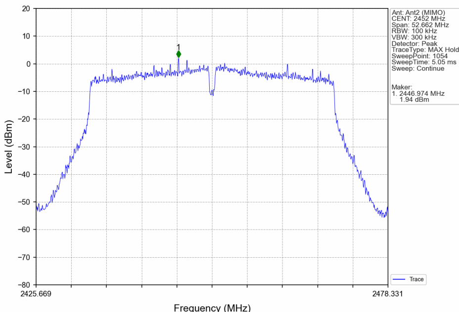
802.11n(HT40)_HCH_2452MHz_Ant2 (MIMO)_NTNV
