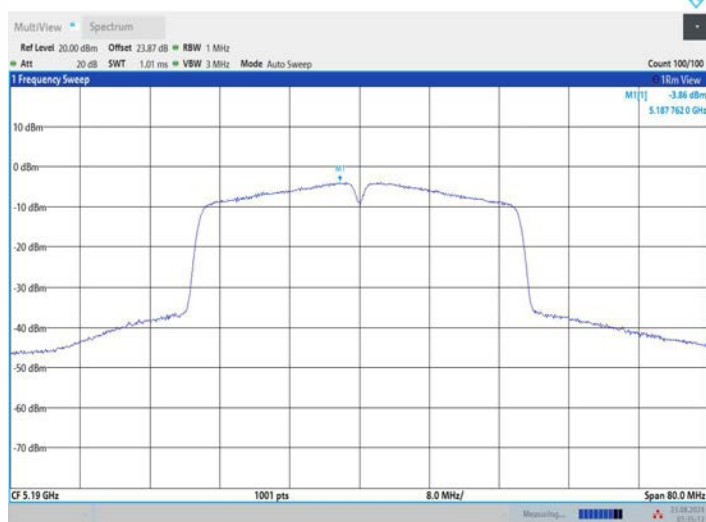
11N40MIMO_Ant3_5190
