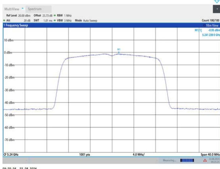
11N20MIMO_Ant3_5240
