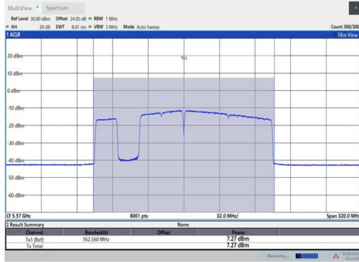
11BE160MIMO_Ant2_5570_996+484+242_OFDMA_2
