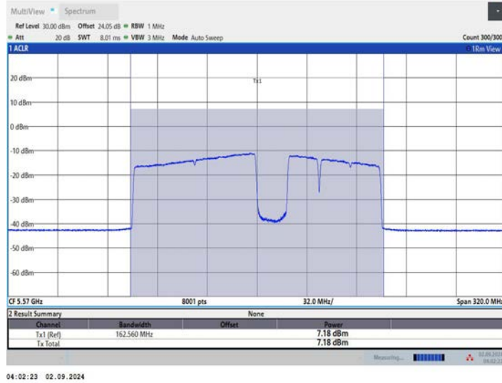
11BE160MIMO_Ant2_5570_996+484+242_OFDMA_5
