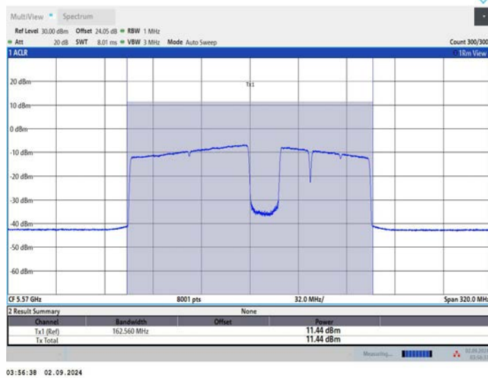
11BE160MIMO_Ant2_5570_996+484+242_OFDMA_6
