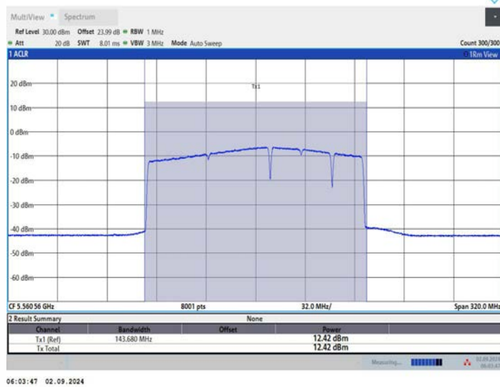
11BE160MIMO_Ant2 5570 996+484 OFDMA 1
