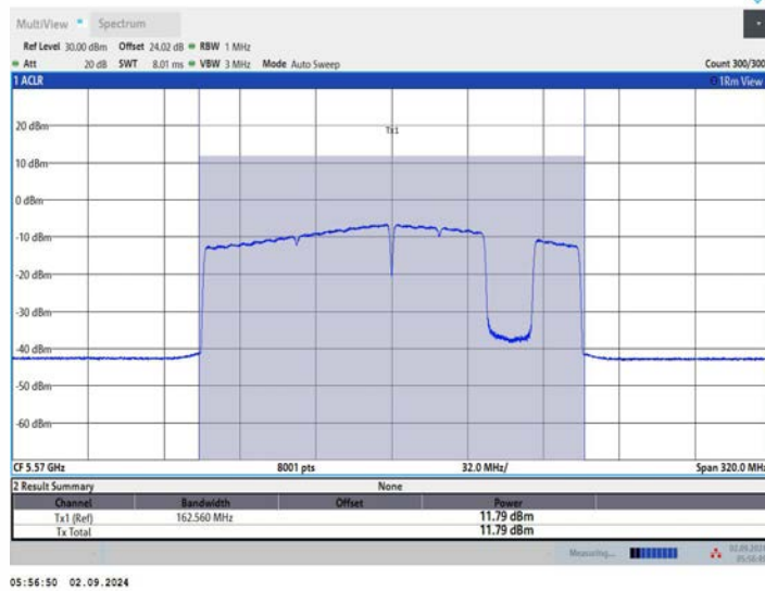
11BE160MIMO_Ant3 5570 996+484+242 OFDMA 8
