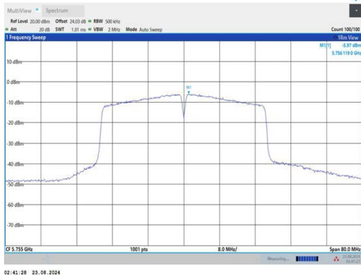
11N40MIMO_Ant3_5755
