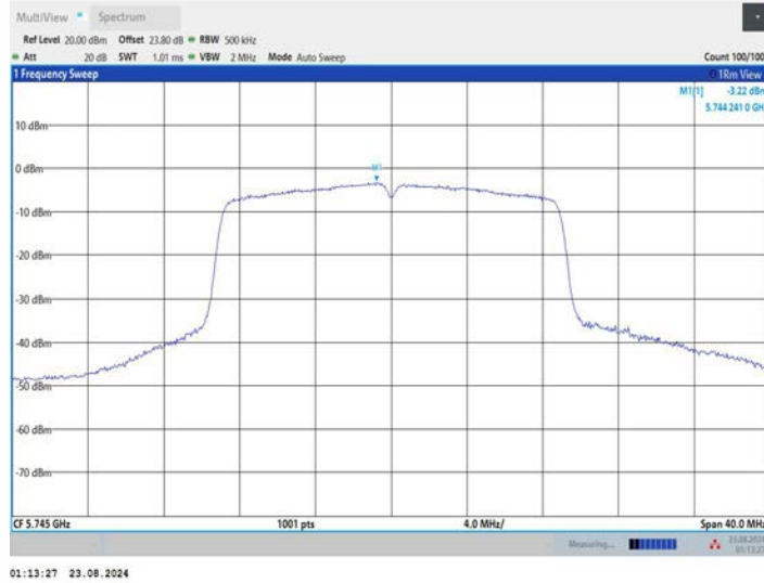
11N20MIMO_Ant3_5745
