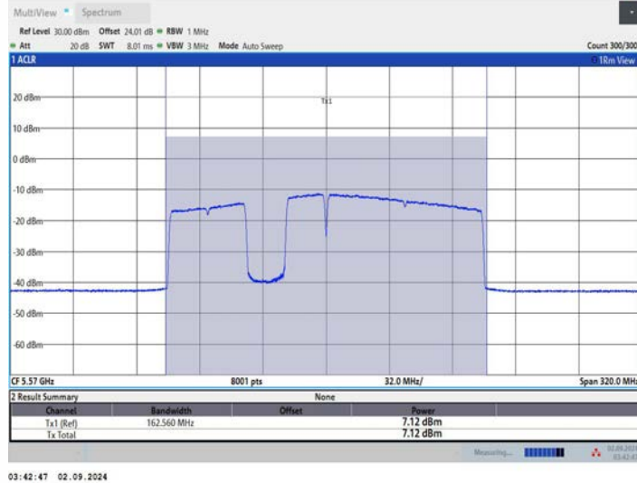
11BE160MIMO_Ant2_5570_996+484+242_OFDMA_3
