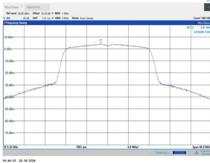
11A_Ant2_5320
