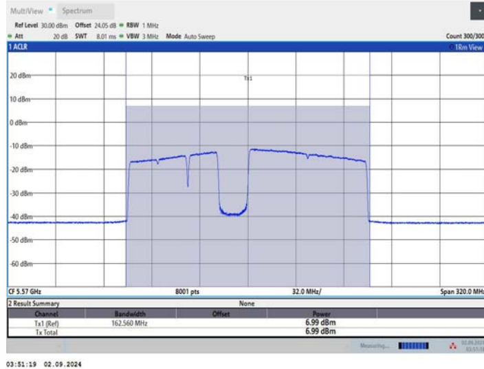
11BE160MIMO_Ant2_5570_996+484+242_OFDMA_4
