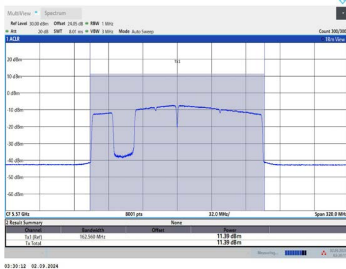
11BE160MIMO_Ant2_5570_996+484+242_OFDMA_3
