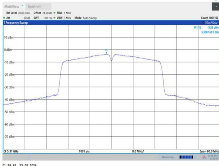
11N40MIMO_Ant3_5310
