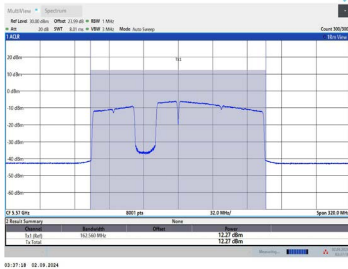
11BE160MIMO_Ant1 5570 996+484+242 OFDMA 4
