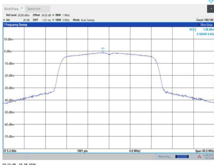
11AC20MIMO_Ant3_5200
