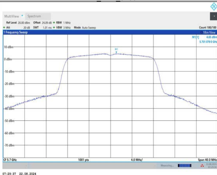
11A_Ant3_5700
