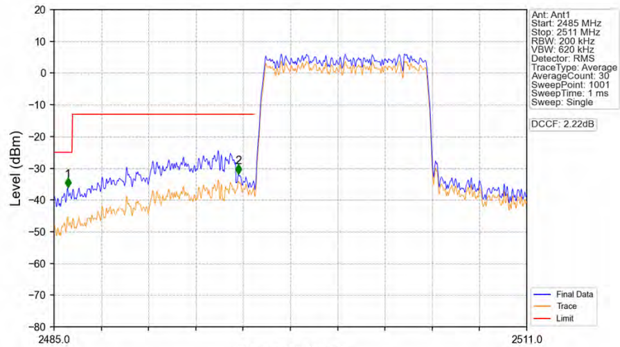
Band41_10MHz_16QAM_LCH_2501MHz_RB_50_0_NTNV
