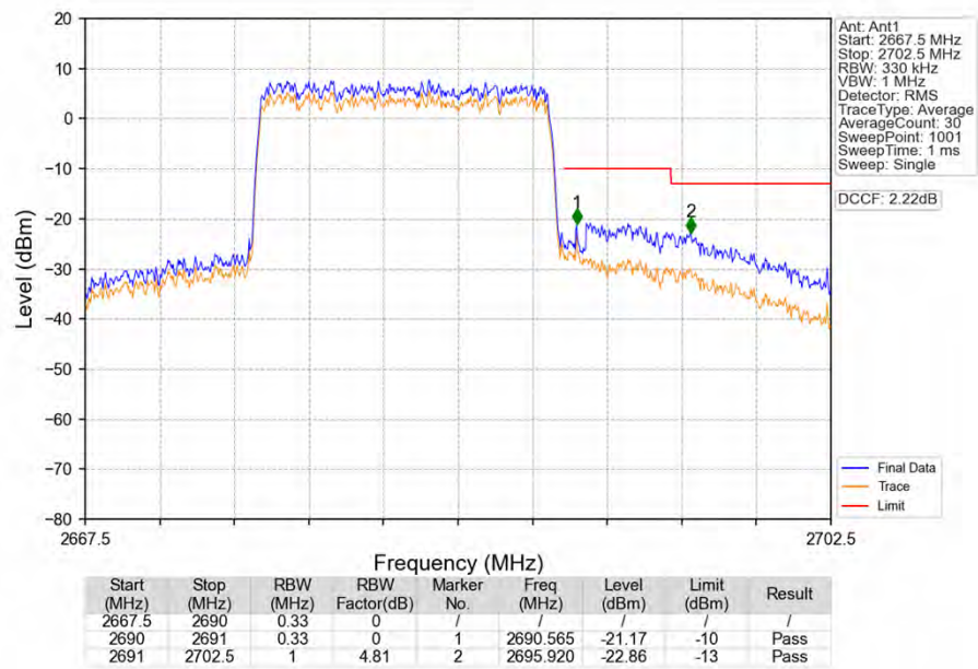
Band41_15MHz_QPSK_HCH_2682.5MHz_RB_75_0_NTNV
