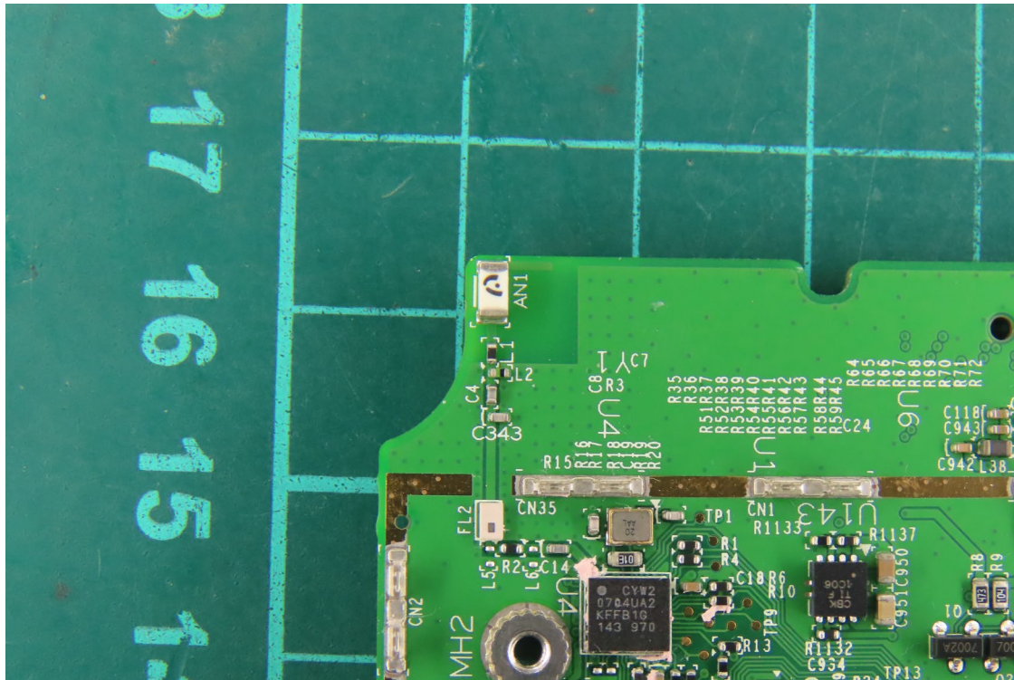
(37) EUT Photo
