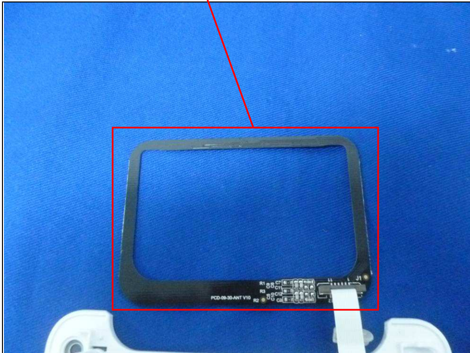
NFC Antenna
