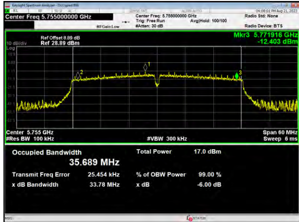
5755MHz
