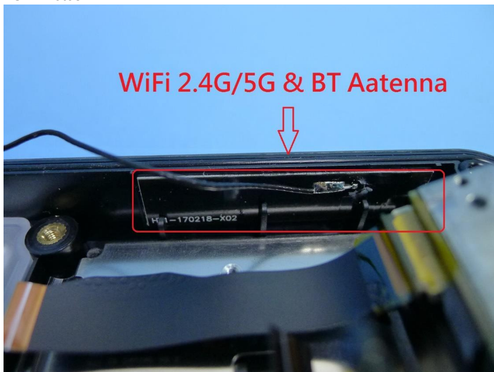
(4) EUT Photos
