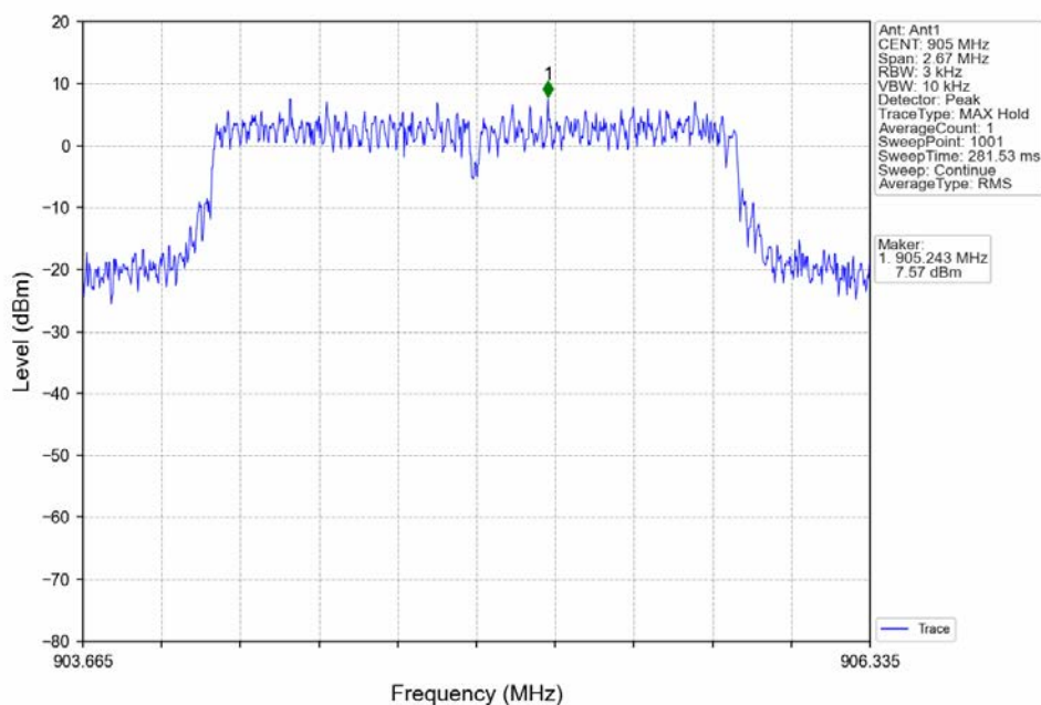
2M_LCH_905MHz_Ant1_NTNV
