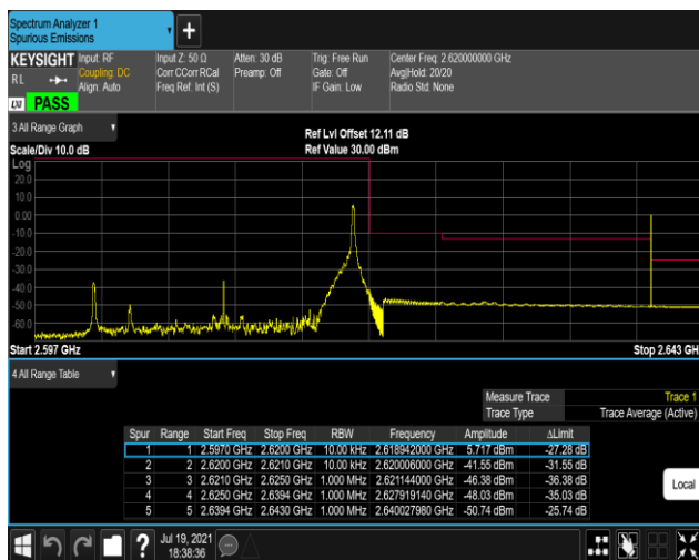
Band38-20MHz-QPSK-38150-1RB#99
