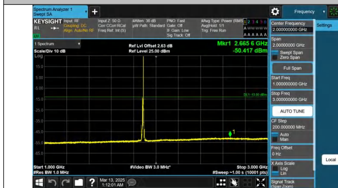
Band25-10MHz-QPSK-26365-1RB#49-1000~3000-PASS
