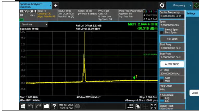
Band25-20MHz-QPSK-26365-1RB#99-1000~3000-PASS
