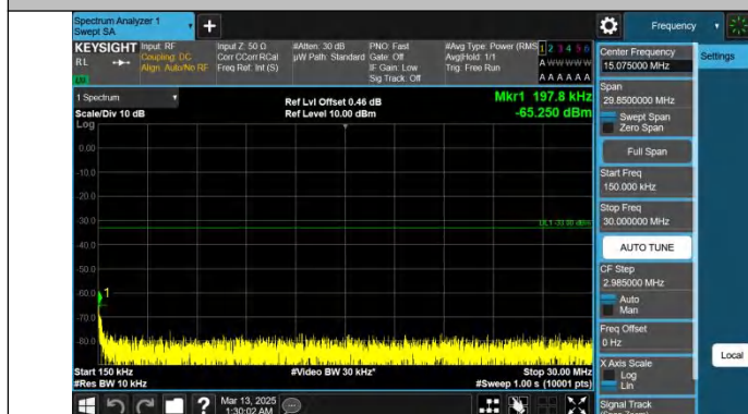
Band25-20MHz-QPSK-26365-1RB#99-0.15~30-PASS
