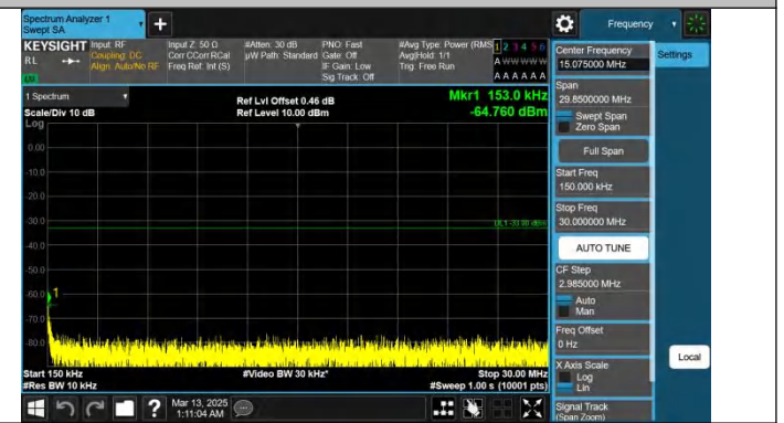
Band25-10MHz-QPSK-26365-1RB#0-0.15~30-PASS
