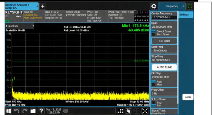
Band25-20MHz-QPSK-26365-1RB#0-0.15~30-PASS
