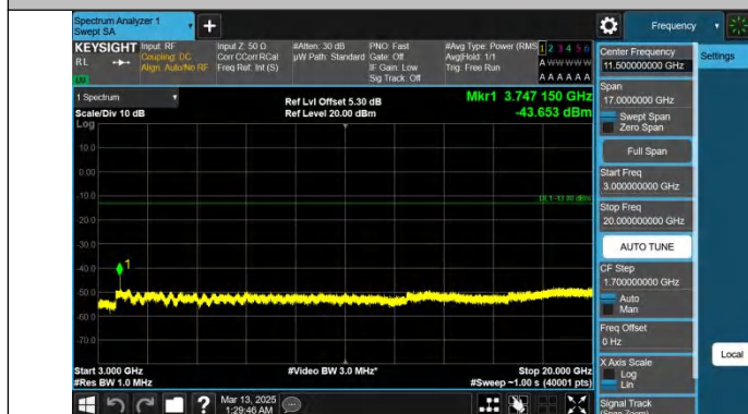
Band25-20MHz-QPSK-26365-1RB#0-3000~20000-PASS
