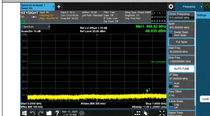
Band25-10MHz-QPSK-26365-1RB#0-30~1000-PASS
