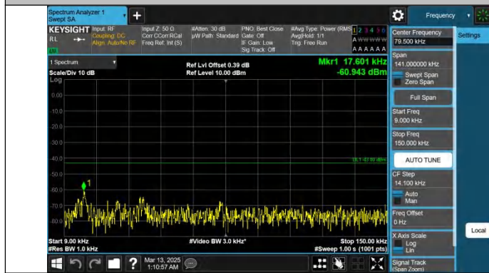
Band25-10MHz-QPSK-26365-1RB#0-0.009~0.15-PASS
