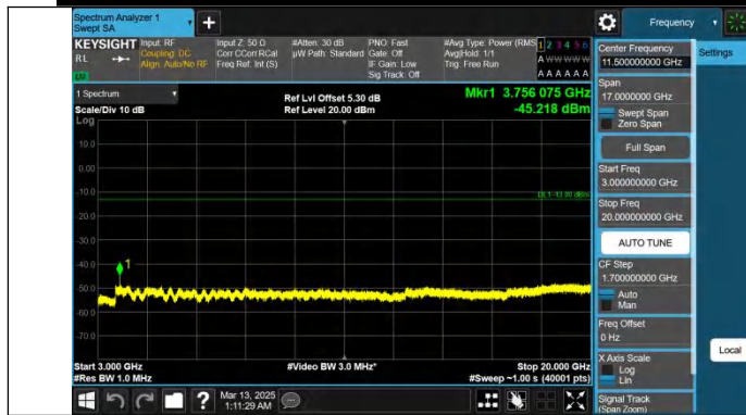
Band25-10MHz-QPSK-26365-1RB#0-3000~20000-PASS
