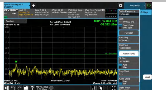
Band25-20MHz-QPSK-26365-1RB#99-0.009~0.15-PASS
