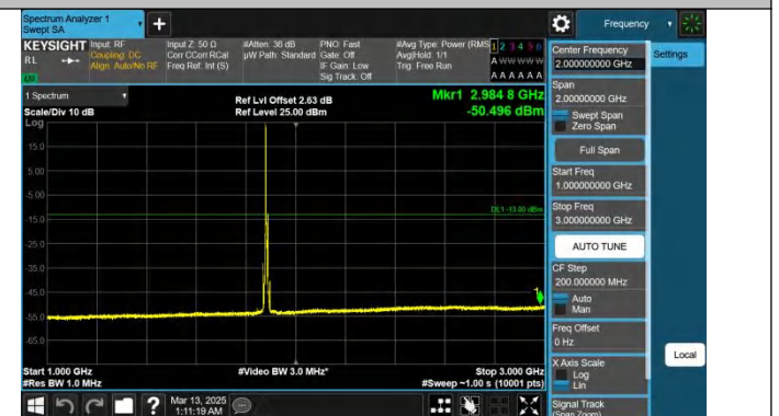
Band25-10MHz-QPSK-26365-1RB#0-1000~3000-PASS
