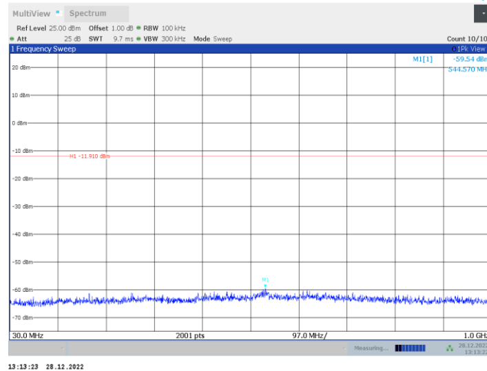
BLE 1M Ant6 2402 30~1000
