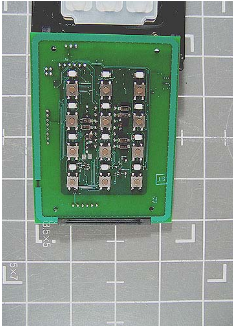
PCB Bottom
