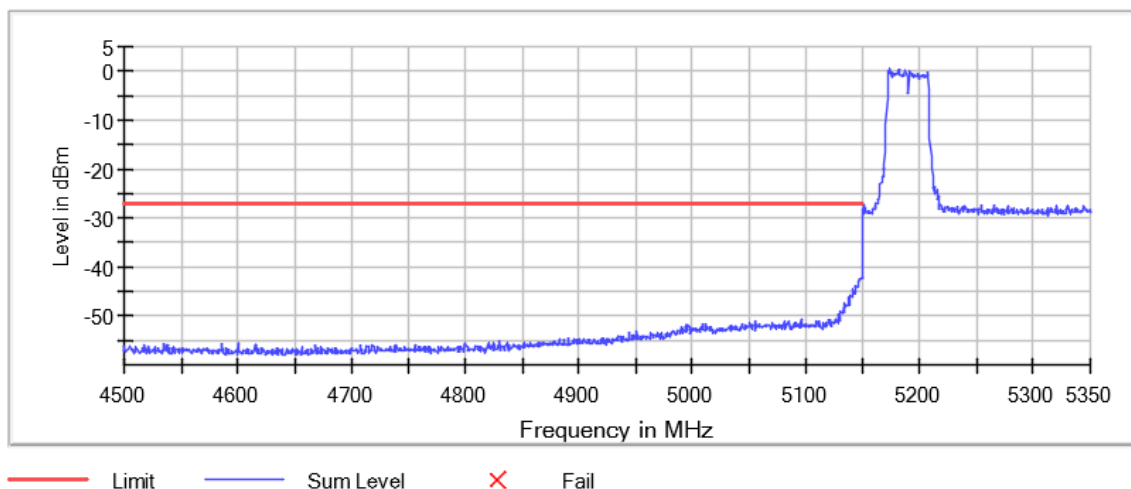
Band Edge
