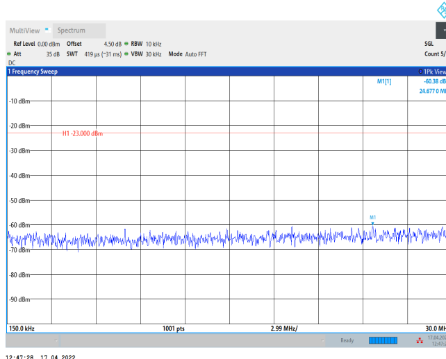
Band26-10MHz-QPSK-26740-1RB#0-Range2:0.15~30MHz
