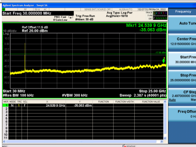
802.11g,2437MHz, Ant1, Plot 2,30MHz~2500 0MHz
