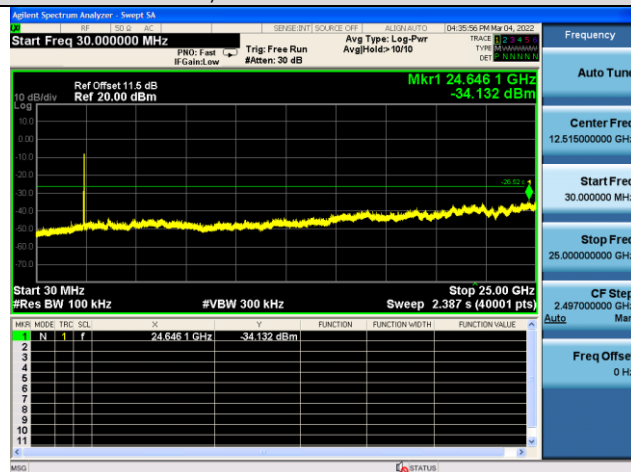
802.11n-HT 20,2437MHz, Ant0, Plot 2, 30MHz~25000MHz
