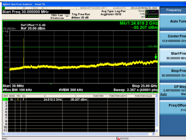
802.11b,2437MHz, Ant0, Plot 2,30MHz~2500 OMHz
