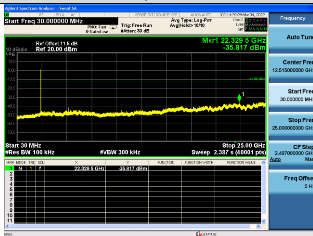
802.11b,2437MHz, Ant1, Plot 2,30MHz~2500 OMHz
