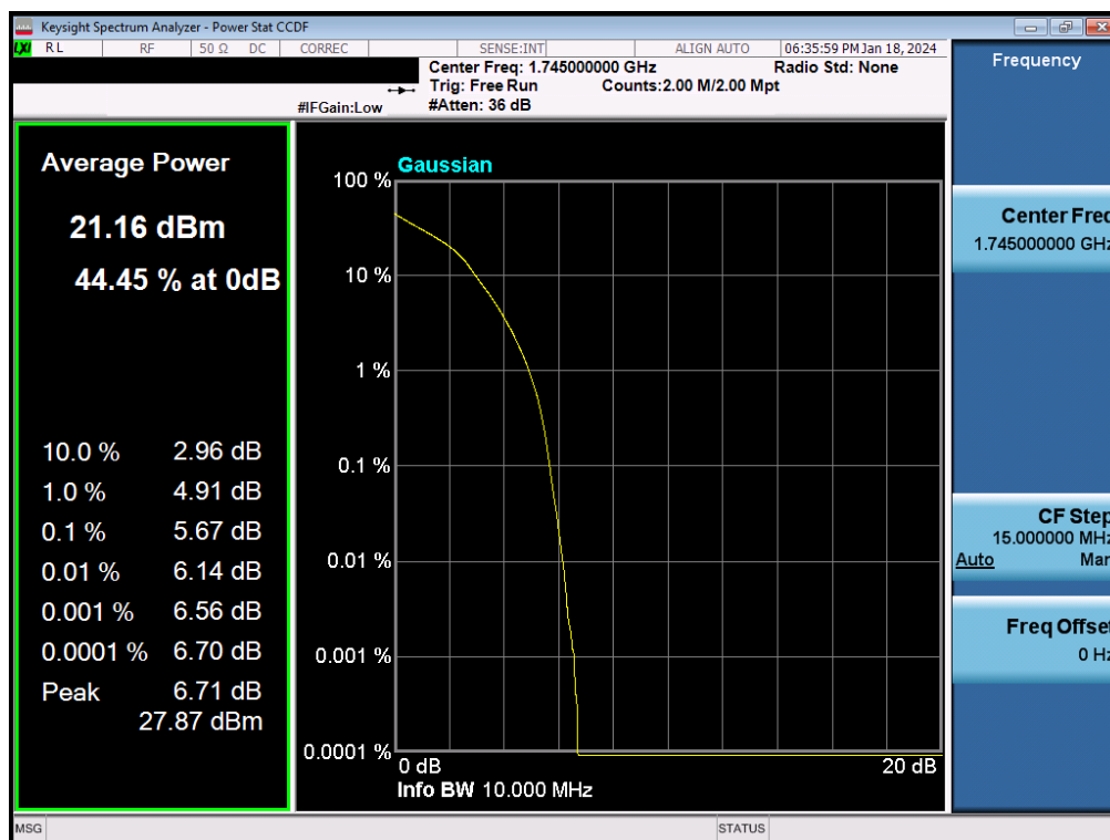
Plot 7-115. PAR Plot (LTE Band 66/4 - 10MHz 16-QAM - Full RB)
