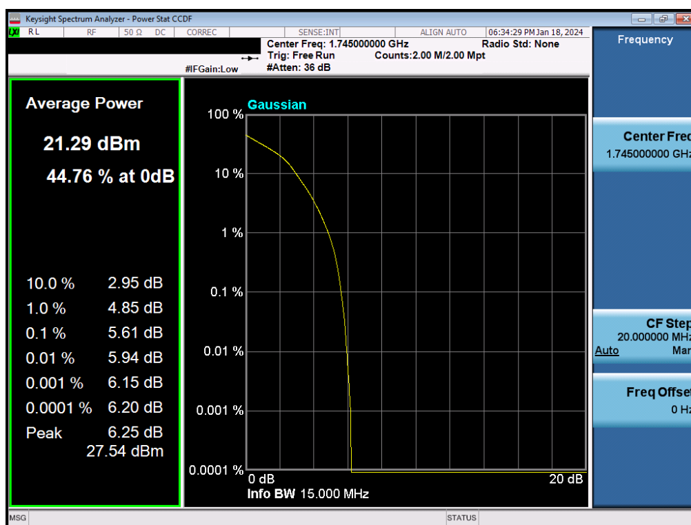
Plot 7-113. PAR Plot (LTE Band 66/4 - 15MHz 16-QAM - Full RB)
