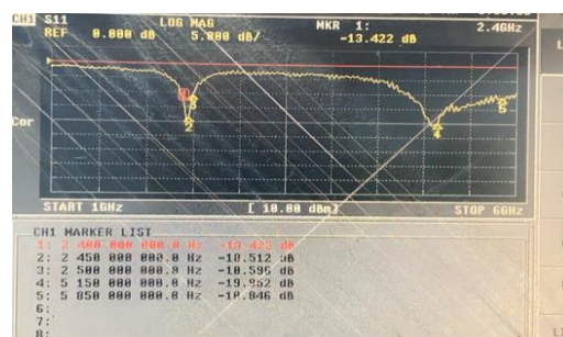
Aux - S11
