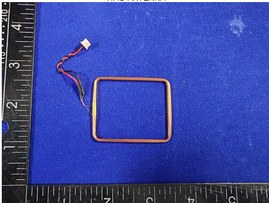
RFID ANTENNA
