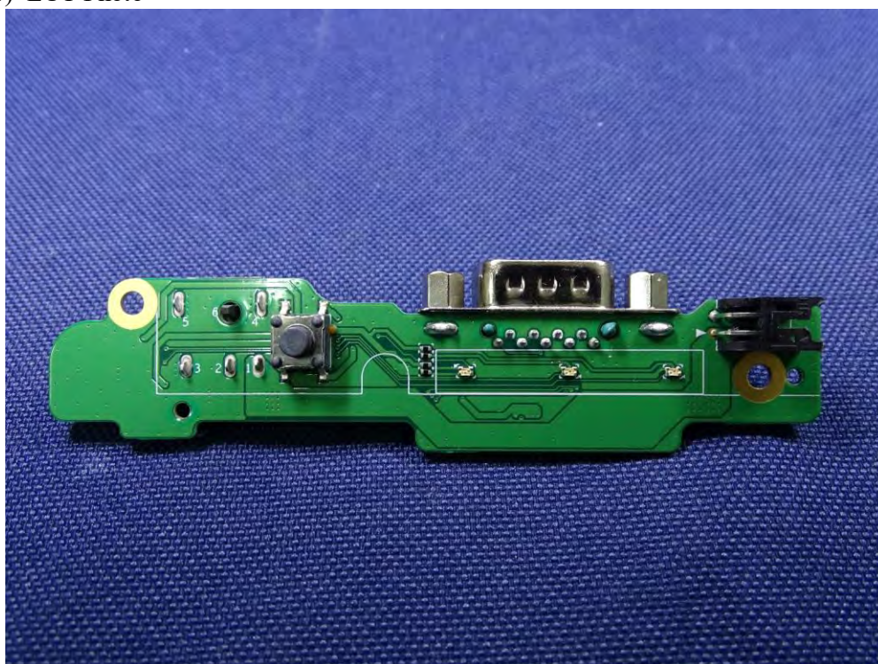
(70) EUT Photo
