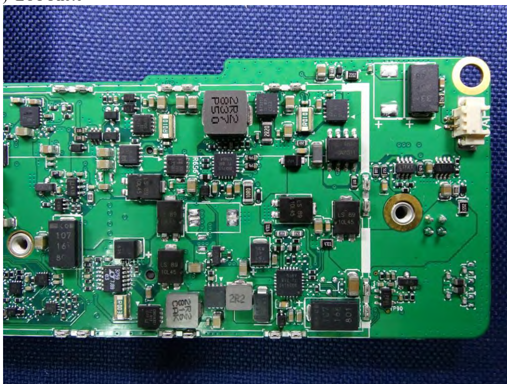
(63) EUT Photo
