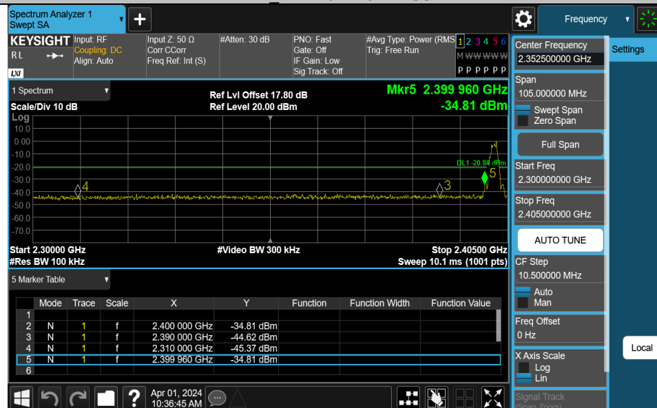
BLE 2M-Ant1-2402-PASS
