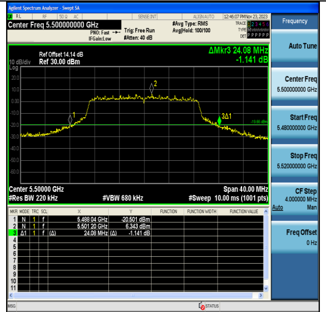
11N20MIMO-Ant7-5500
