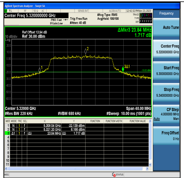
11N20MIMO-Ant7-5320
