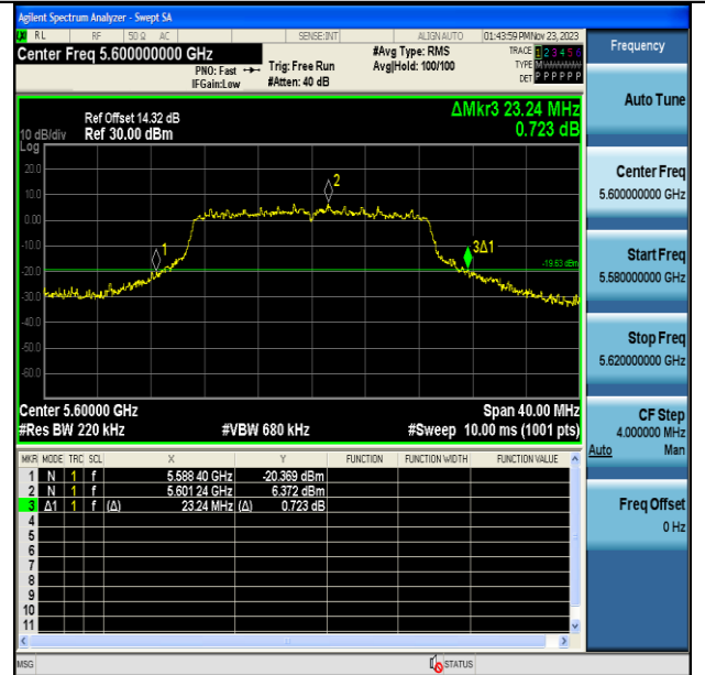
11N20MIMO-Ant7-5600
