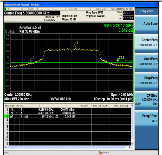
11N20MIMO-Ant7-5300
