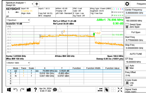
11be EHT80 MID CHANNEL TX0 6dB Bandwidth
