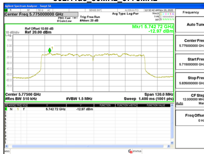
802.11ac_80MHz_5775MHz
