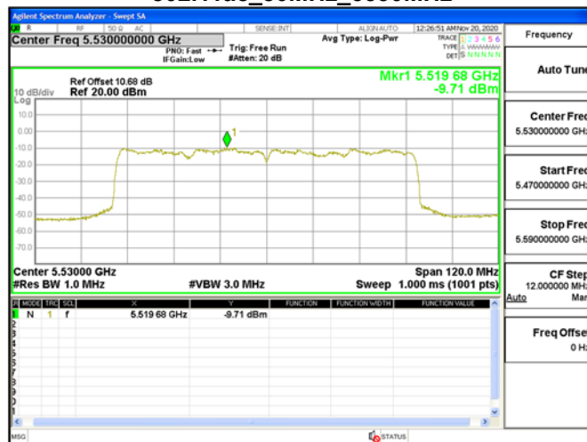
802.11ac_80MHz_5530MHz
