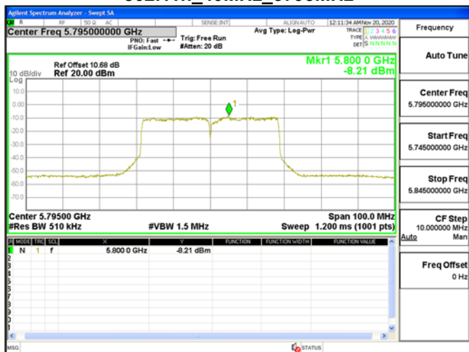
802.11n_40MHz_5795MHz
