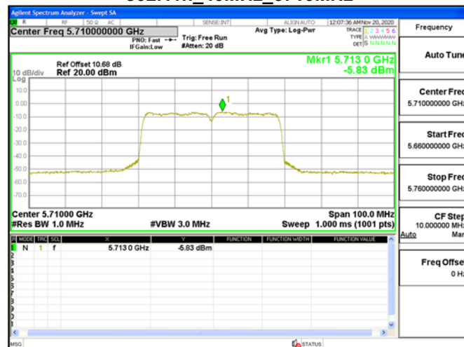
802.11n_40MHz_5710MHz
