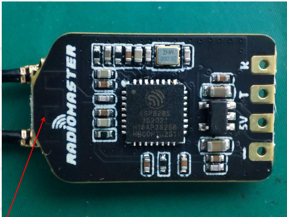
2.4GWIFI ANT
