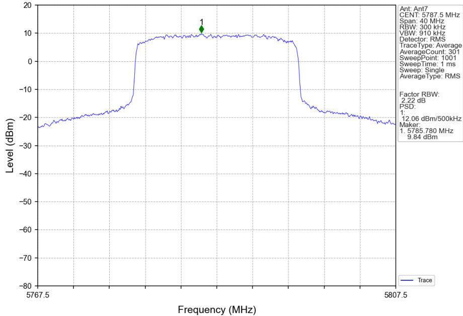
20M_MCH_5787.5MHz_MIMO_NTNV
