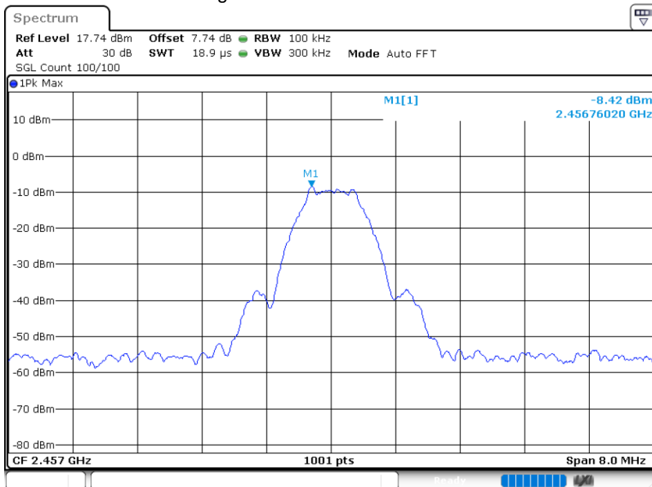
Band Edge NVNT ANT+ 2457MHz Ant1 Ref
