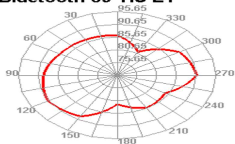
Bluetooth 39 TIS E1
