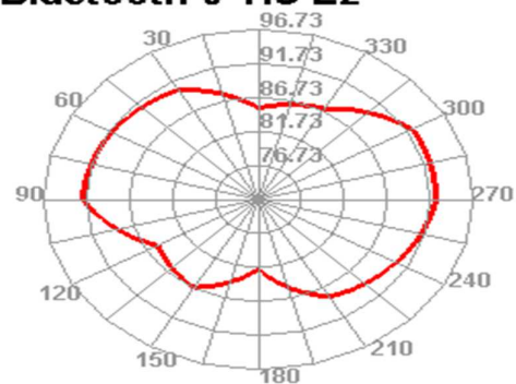
Bluetooth 0 TIS E2
