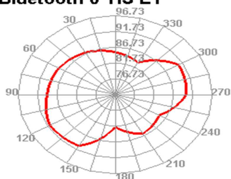
Bluetooth 0 TIS E1
