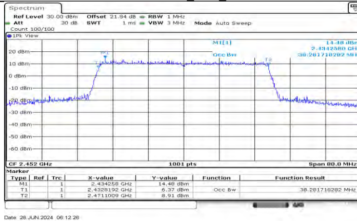
11AX40SISO_Ant1_2452
