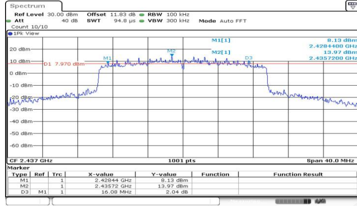
11AX20-CDD_Ant2_2437
