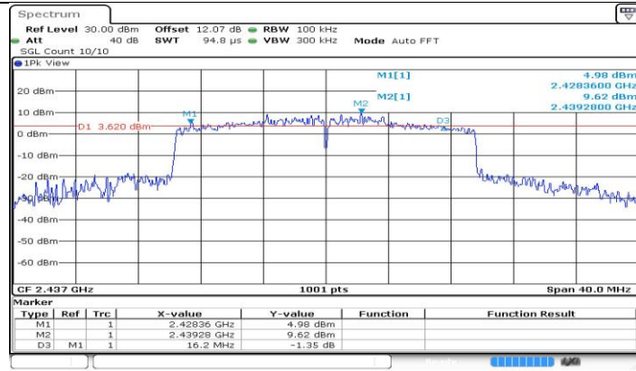
11AX20-CDD_Ant1_2437
