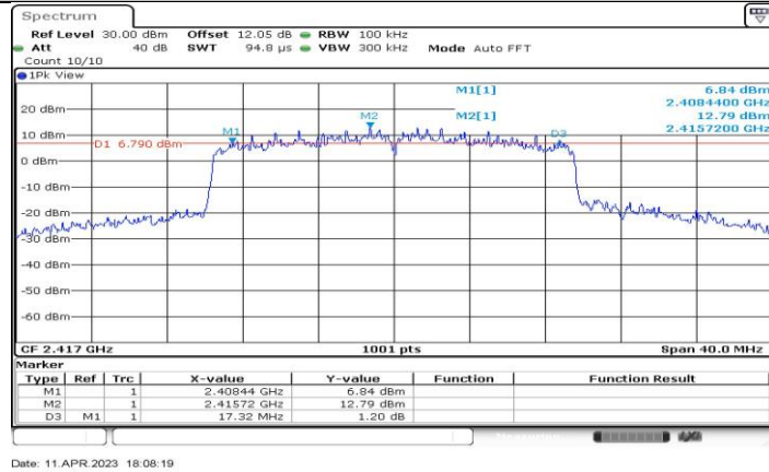
11AX20-CDD_Ant1_2417
