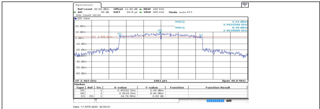
11BE20-CDD_Ant4_2462
