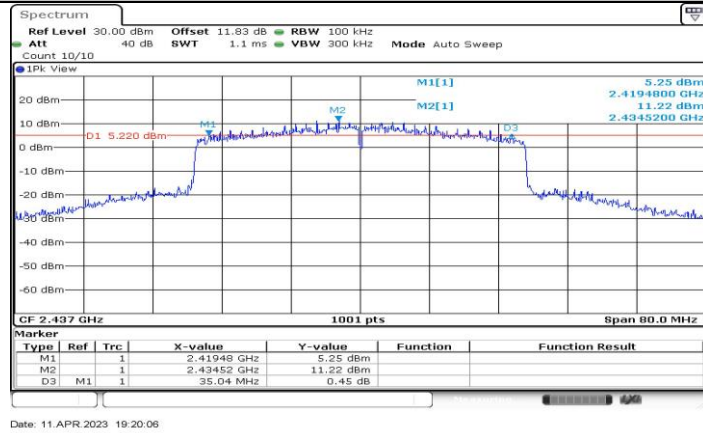
11AX40-CDD_Ant3_2437
