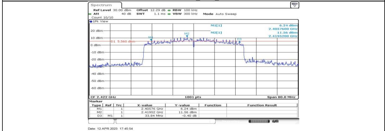
11BE40-CDD_Ant2_2422
