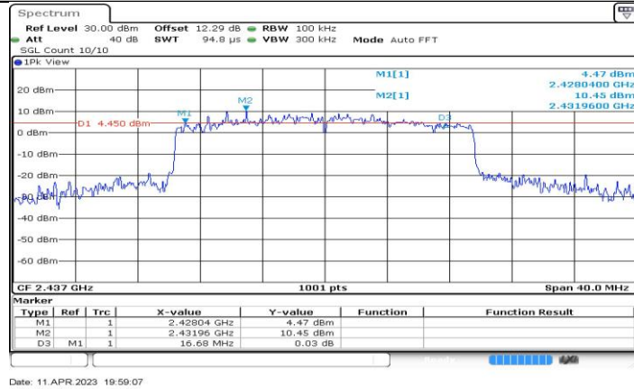
11BE20-CDD_Ant2_2437
