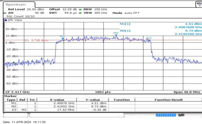
11AX20-CDD_Ant2_2417
