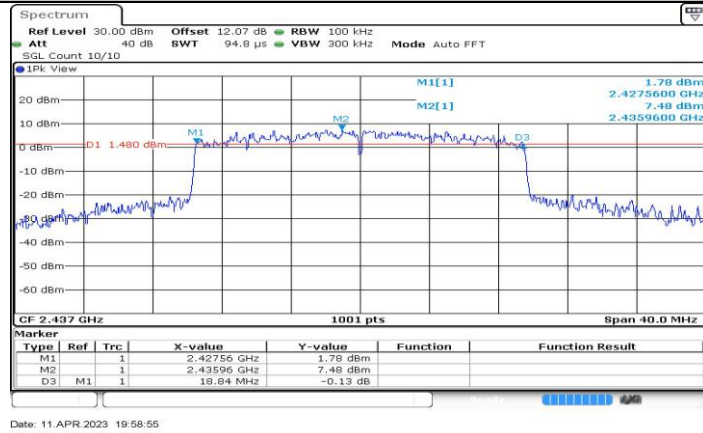
11BE20-CDD_Ant1_2437
