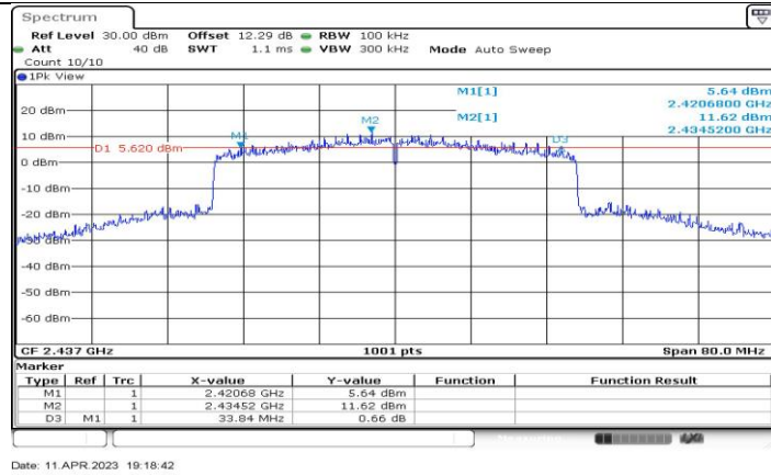
11AX40-CDD_Ant2_2437
