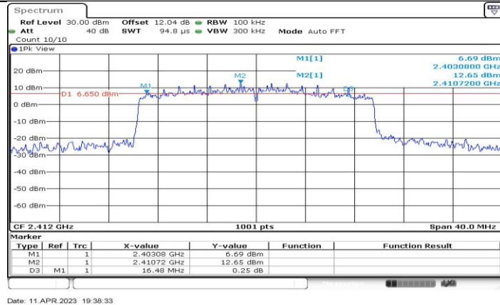
11BE20-CDD_Ant1_2412
