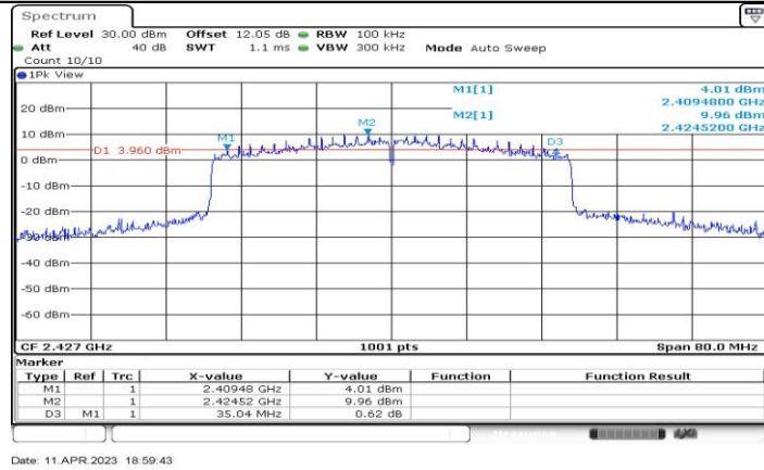
11AX40-CDD_Ant1_2427
