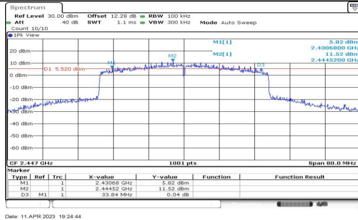
11AX40-CDD_Ant2_2447
