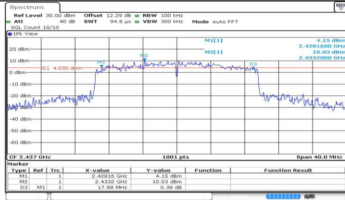
11AX20-CDD_Ant1_2437
