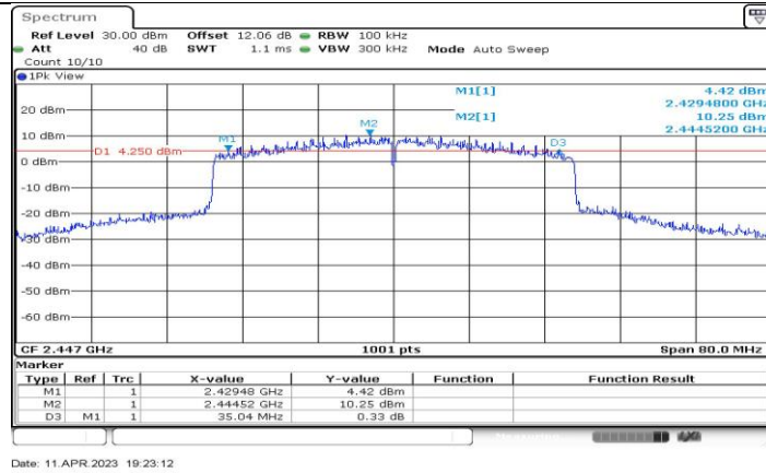
11AX40-CDD_Ant1_2447
