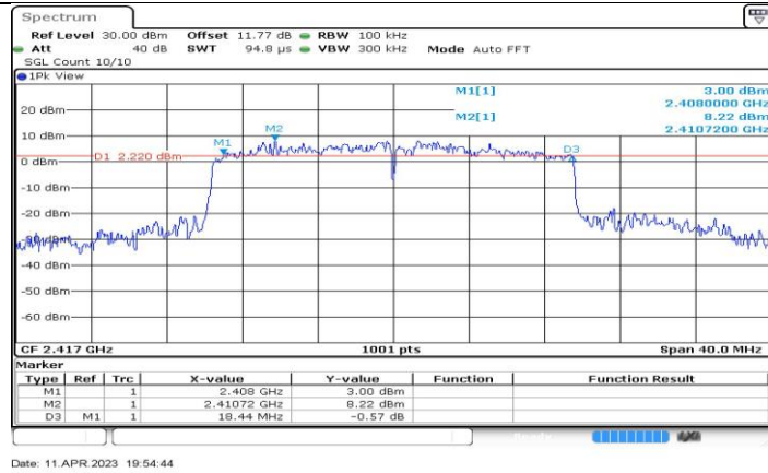
11BE20-CDD_Ant4_2417
