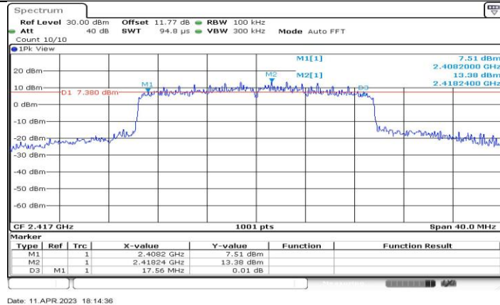
11AX20-CDD_Ant4_2417
