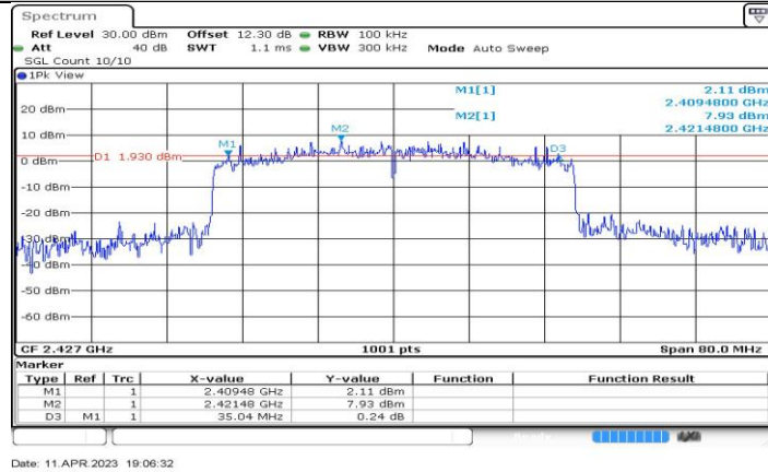
11AX40-CDD_Ant2_2427
