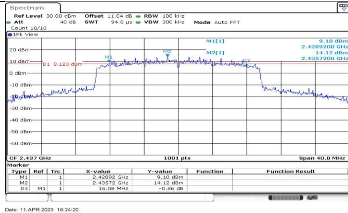
11AX20-CDD_Ant4_2437
