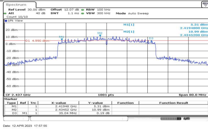
11BE40-CDD_Ant1_2437
