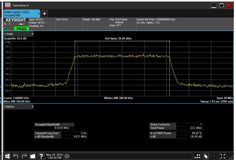
10MHz_30kHz_3840MHz_DFT-s-OFDM QPSK_RB24@0
