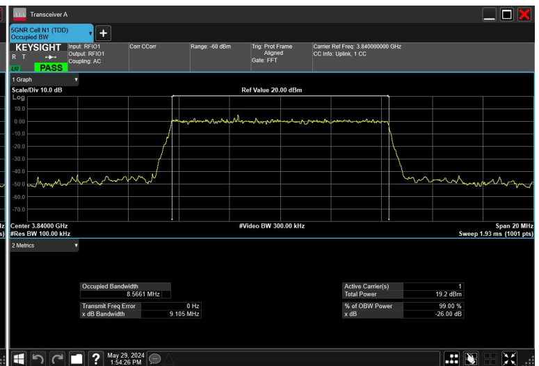
10MHz_30kHz_3840MHz_CP-OFDM QPSK_RB24@0
