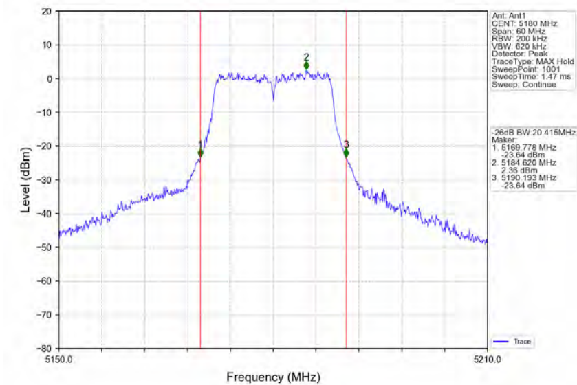
802.11n(HT20)_LCH_5180MHz_Ant1_NTNV
