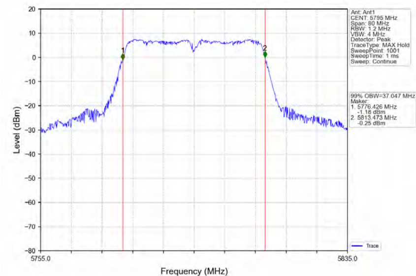
802.11n(HT40)_HCH_5795MHz_Ant1_NTNV
