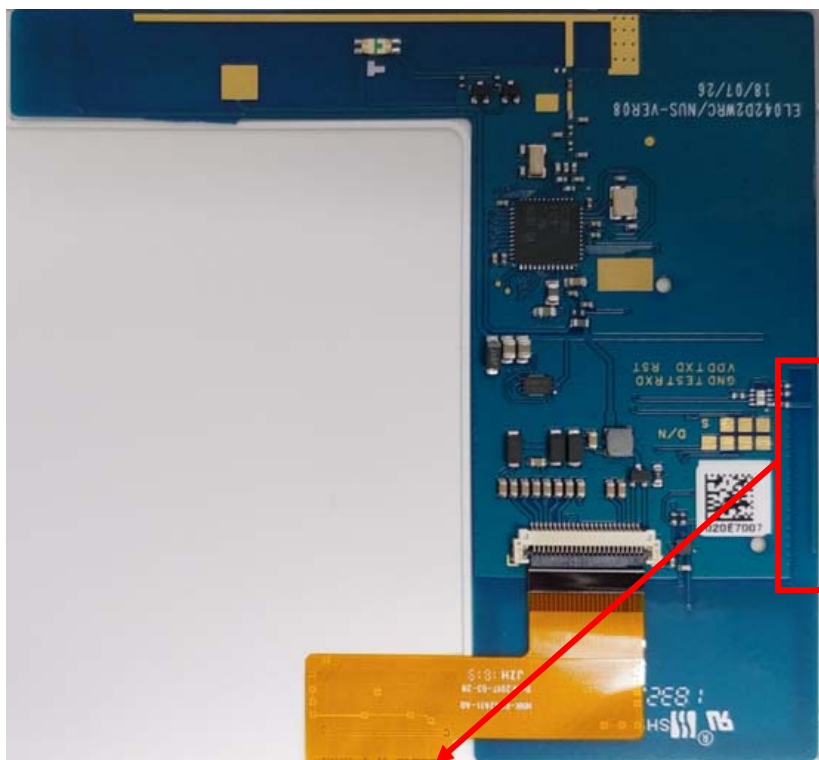
Wake up Antenna(RX)
