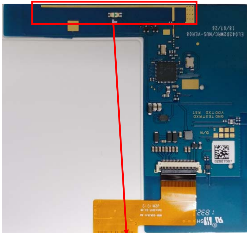
Zigbee Antenna(TX, RX)
