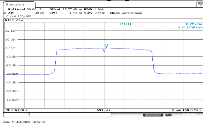
11AC80MIMO_Ant3_5610
