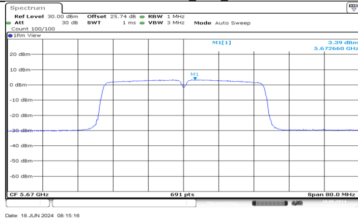
11AC40MIMO_Ant3_5670
