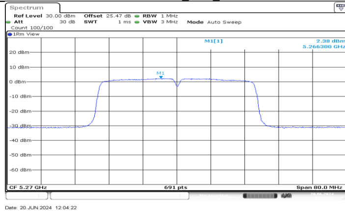
11AC40MIMO_Ant4_5270
