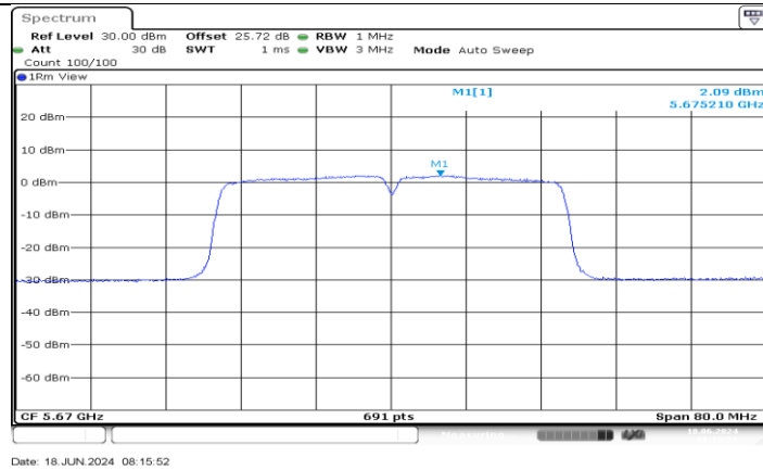
11AC40MIMO_Ant4_5670
