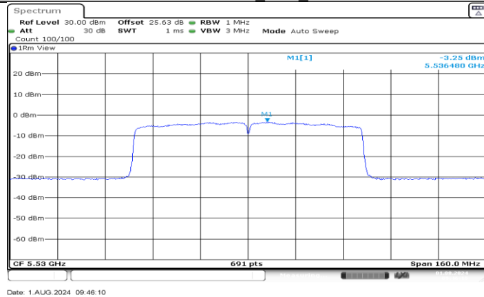
11AC80MIMO_Ant4_5530
