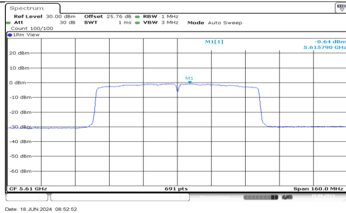
11AC80MIMO_Ant4_5610
