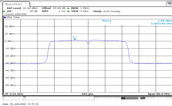
11AC40MIMO_Ant1_5310
