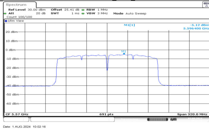
11AC160MIMO_Ant4_5570
