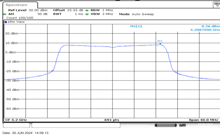
11AX20MIMO_Ant3_5200
