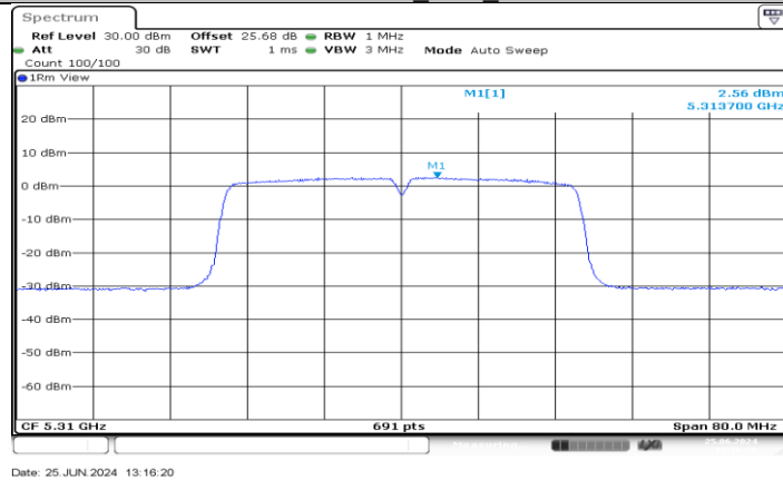
11AC40MIMO_Ant3_5310
