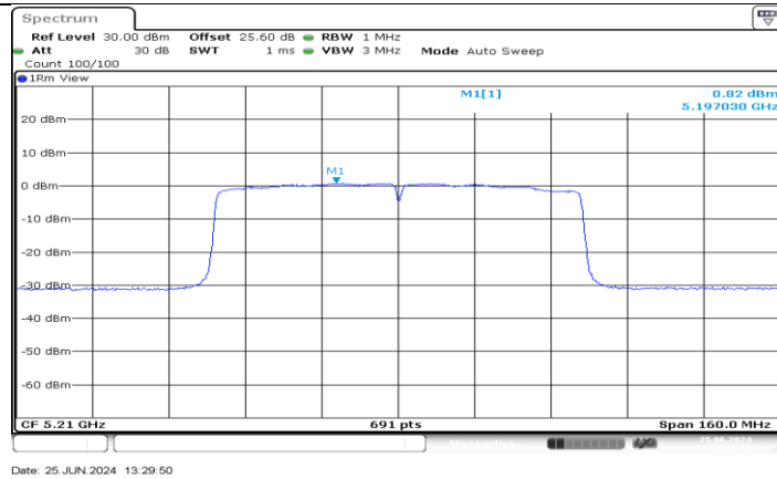
11AC80MIMO_Ant4_5210
