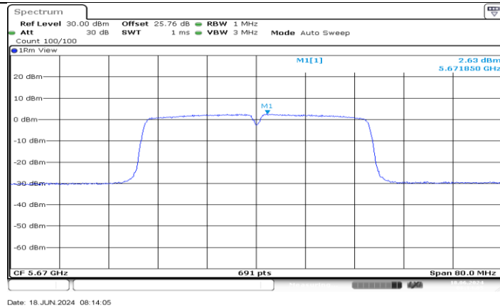
11AC40MIMO_Ant1_5670
