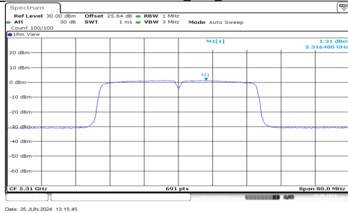
11AC40MIMO_Ant2_5310
