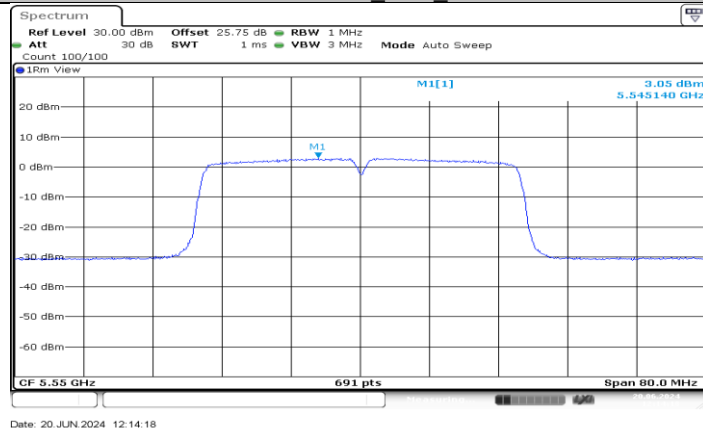
11AC40MIMO_Ant3_5550
