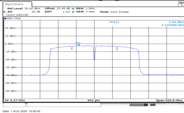
11AC160MIMO_Ant2_5570
