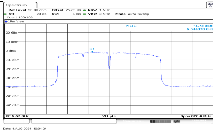
11AC160MIMO_Ant3_5570
