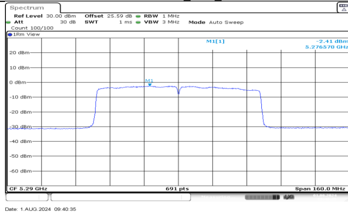
11AC80MIMO_Ant4_5290
