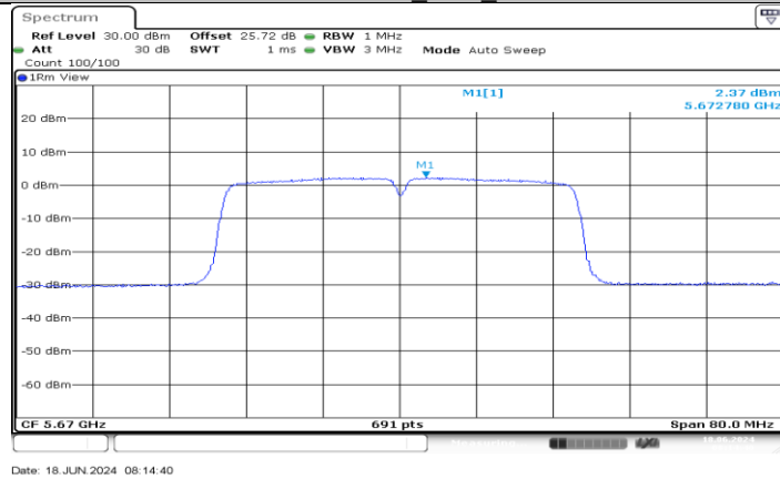
11AC40MIMO_Ant2_5670
