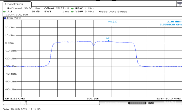
11AC40MIMO_Ant4_5550
