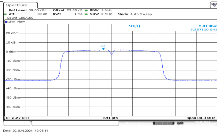
11AC40MIMO_Ant2_5270
