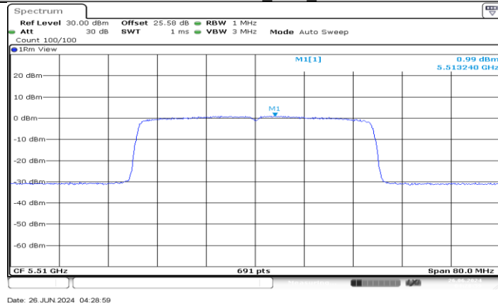
11AX40MIMO_Ant3_5510
