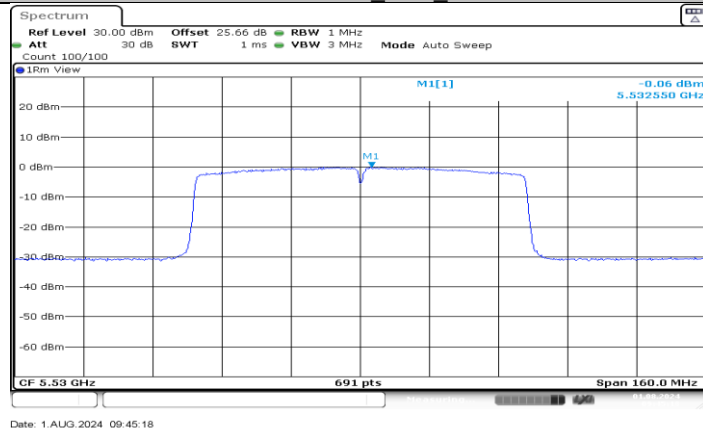
11AC80MIMO_Ant3_5530
