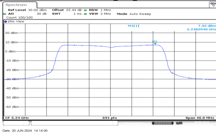
11AX20MIMO_Ant4_5240
