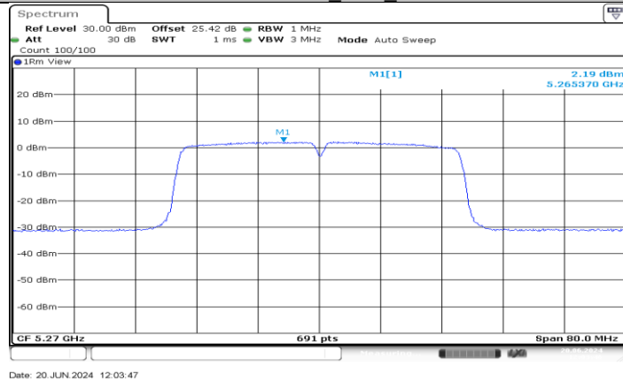
11AC40MIMO_Ant3_5270
