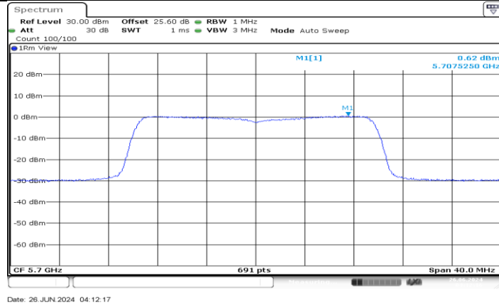
11AX20MIMO_Ant4_5700
