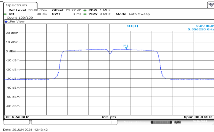
11AC40MIMO_Ant2_5550
