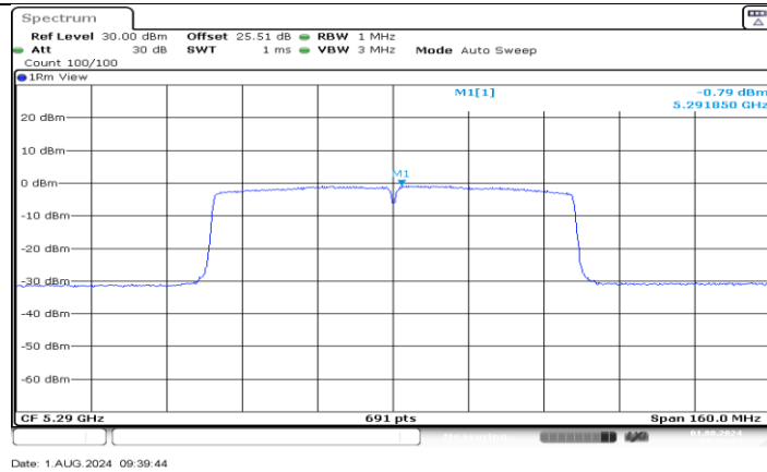
11AC80MIMO_Ant3_5290
