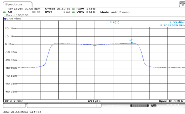
11AX20MIMO_Ant3_5700
