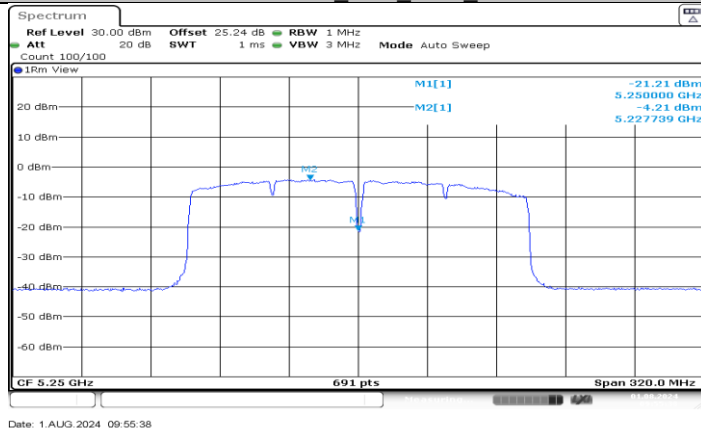
11AC160MIMO_Ant4_5250_UNII-1
