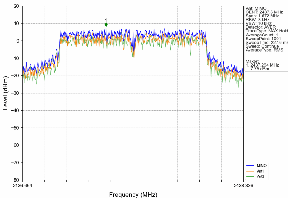
1.4M_MCH_2437.5MHz_MIMO_NTNV
