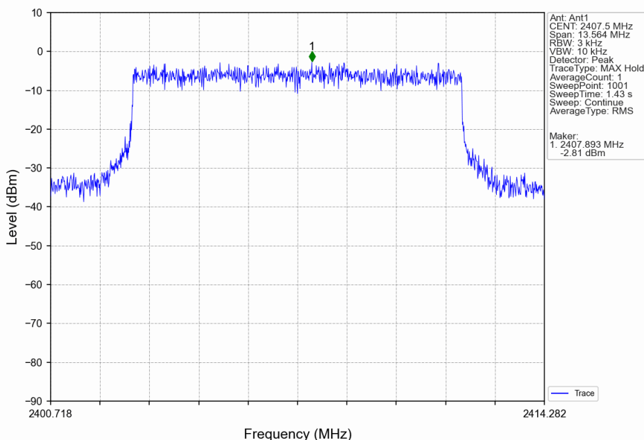
10M_LCH_2407.5MHz_MIMO_NTNV
