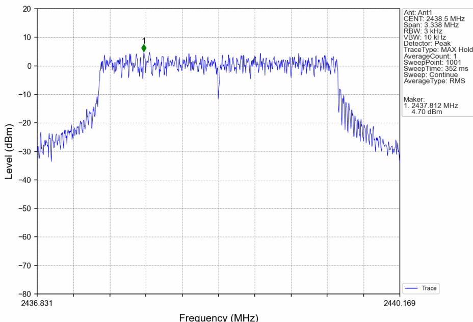
3M_MCH_2438.5MHz_Ant1_NTNV
