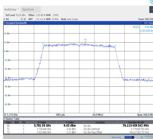
11ac80SISO-Ant23-5775
