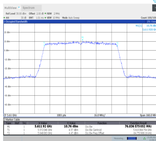
11ac80SISO-Ant23-5610
