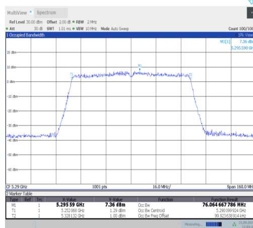
11ac80SISO-Ant23-5290
