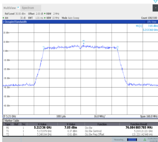
11ac80SISO-Ant23-5210
