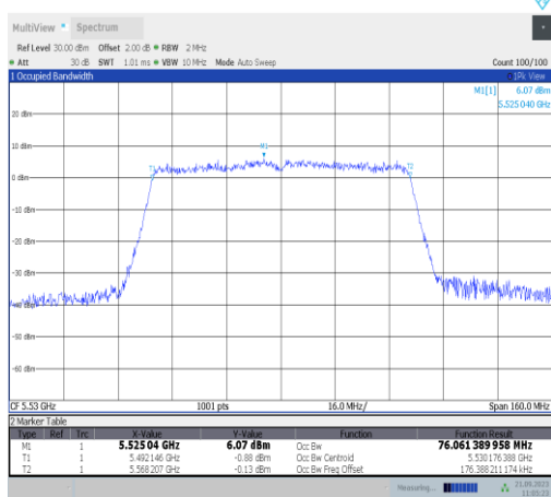
11ac80SISO-Ant23-5530
