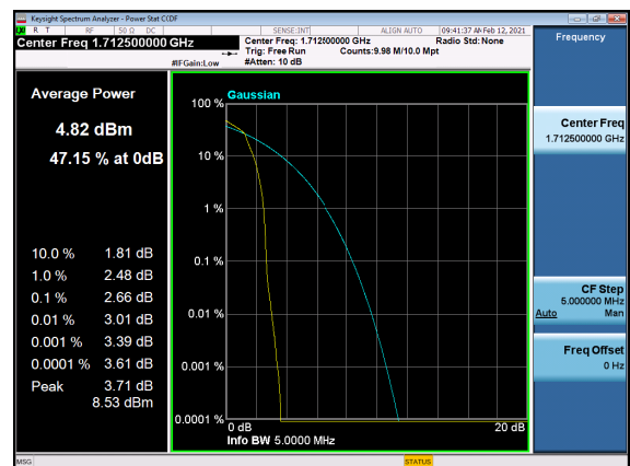
B2_N66(5M)_DFT-s-OFDM_BPSK_Edge_1R B_Left_Low_CH
