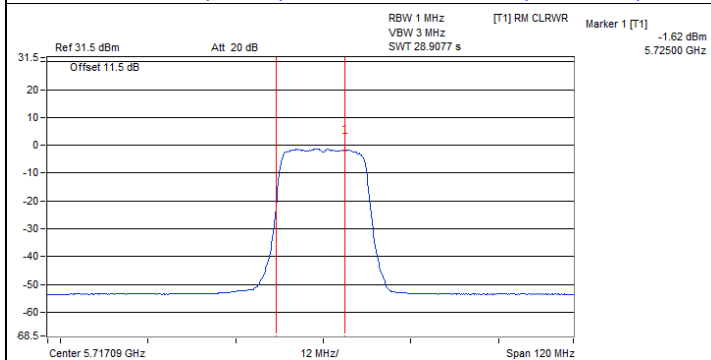
802.11ax (HE20) / Chain 2 : CH 144 (U-NII-2C)
