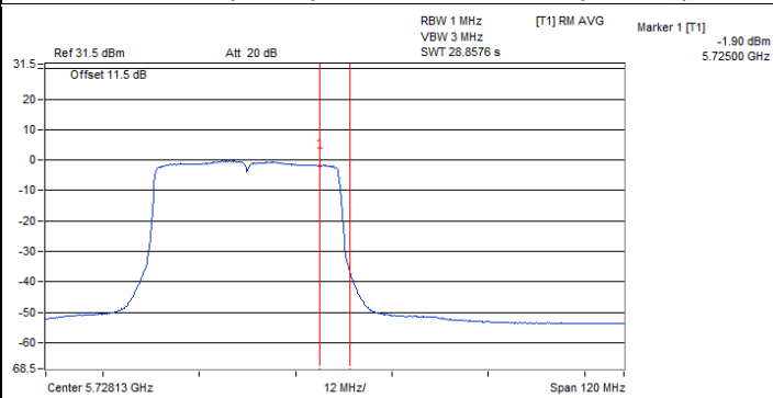
802.11ax (HE20) / Chain 3 : CH 144 (U-NII-3)
