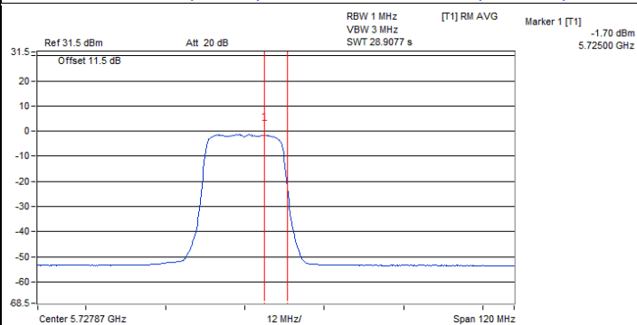
802.11ax (HE20) / Chain 2 : CH 144 (U-NII-3)
