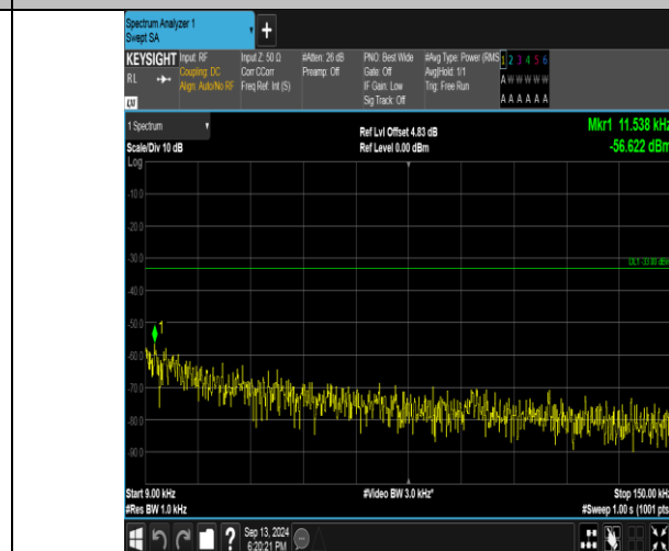
Band26 1.4MHz 16QAM 26915 1RB#0 0.009~0.15 0.009~0.15
