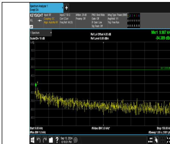
Band26 1.4MHz QPSK 26915 1RB#0 0.009~0.15 0.009~0.15
