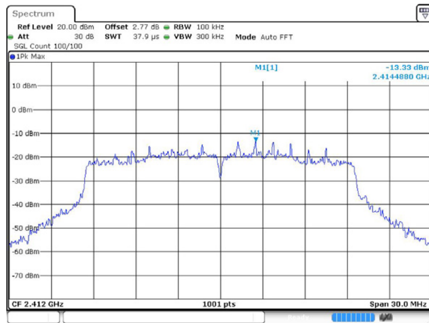
ax20 2412MHz Ant1 Ref
