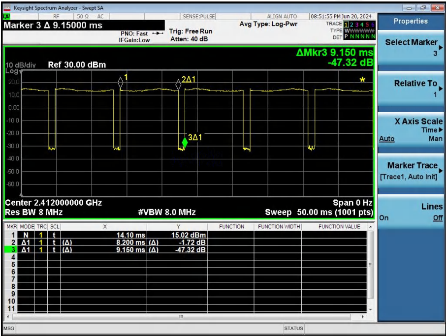
802.11b 2412MHz
