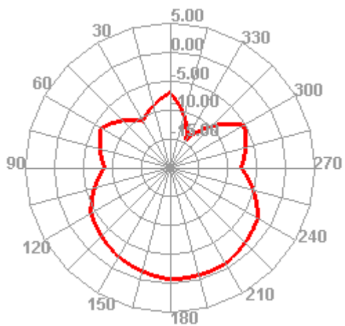
5G phi=0deg
