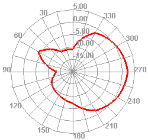
2.4G theta=90deg
