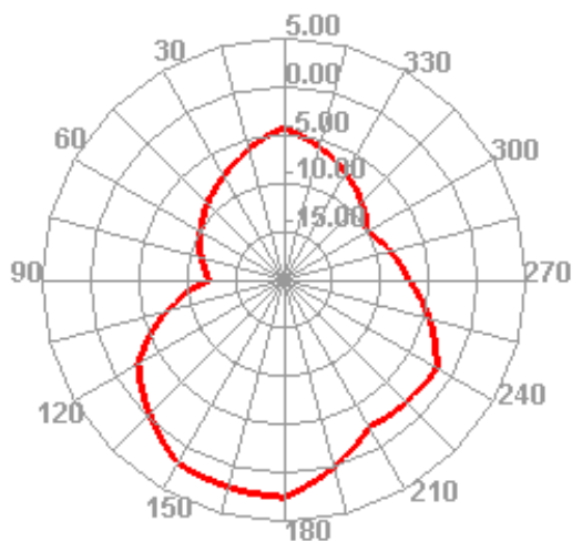
2.4G phi=0deg
