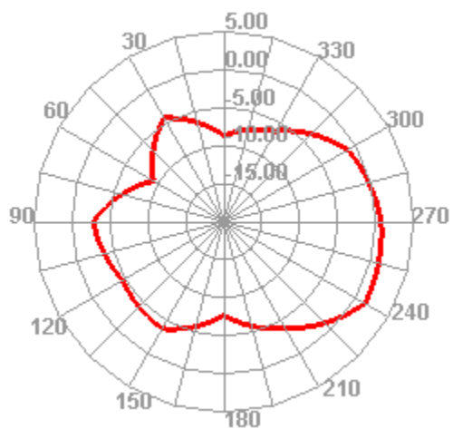
5G theta=90deg
