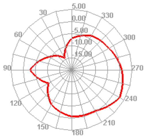
5G phi=90deg
