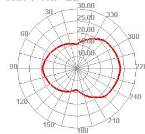
Wifi 1 TRP E2
