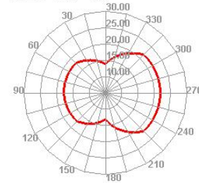
Wifi 7 TRP E2
