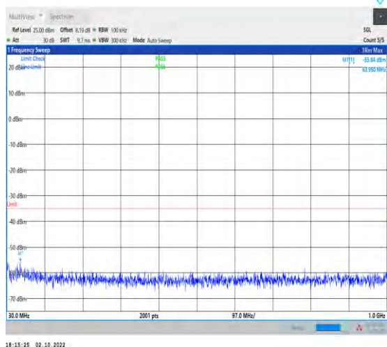
1-N7--15-50-M-1-DFT-PI2BPSK-Inner_1RB_Left-1 @ 1-30-1000-Ant1-63.95--55.84--35-PASS
