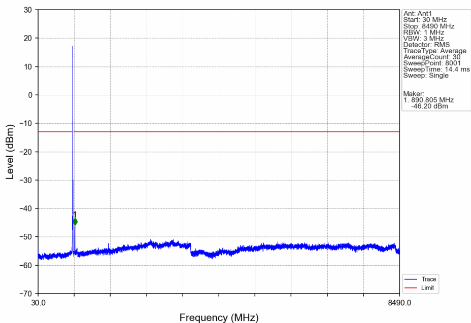
Band5_10MHz_QPSK_HCH_844MHz_RB_1_0 NTN
