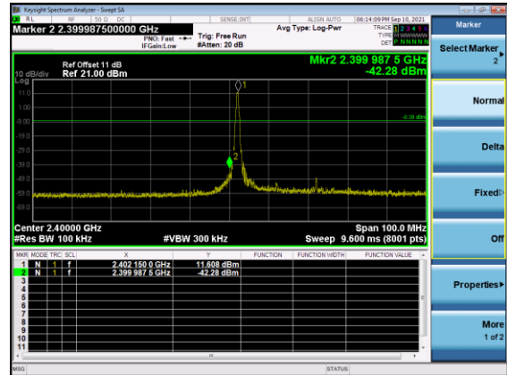
BT GFSK CH00 + 5G 11ac80 CH138
