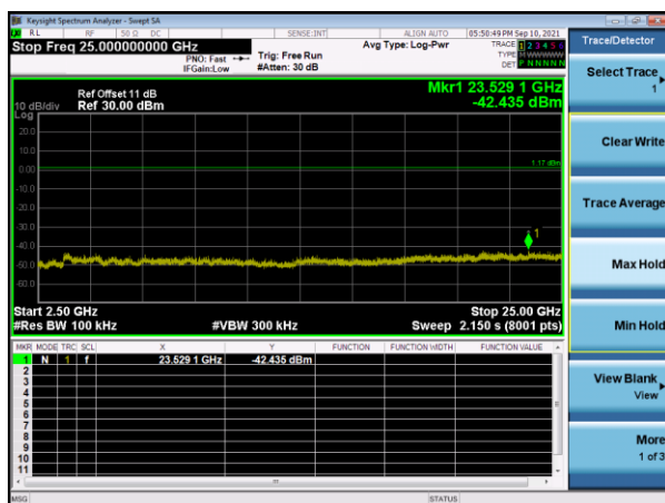
BT GFSK CH00 + 2.4G 11n40 CH09
